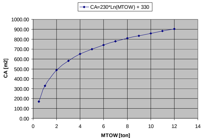
Figuur 18 Oppervlakte van ongevalgevolgebied als functie van MTOW.
