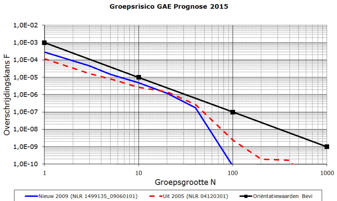
Figuur 13 Groepsrisico (FN-curve) van prognose 2015, vergeleken met resultaat uit het onderzoek van 2005.
