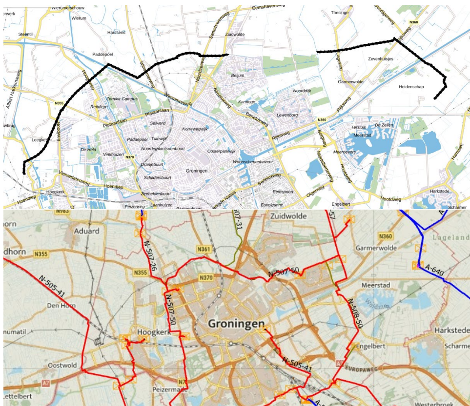
Afbeelding 1, ligging regionale gastransportleidingen (rode lijnen) en hoofd gastransportleidingen (donkerblauw) in en nabij plangebied ontwerp TAM-omgevingsplan 110kV-kabelverbinding Vierverlaten-Meerstad
