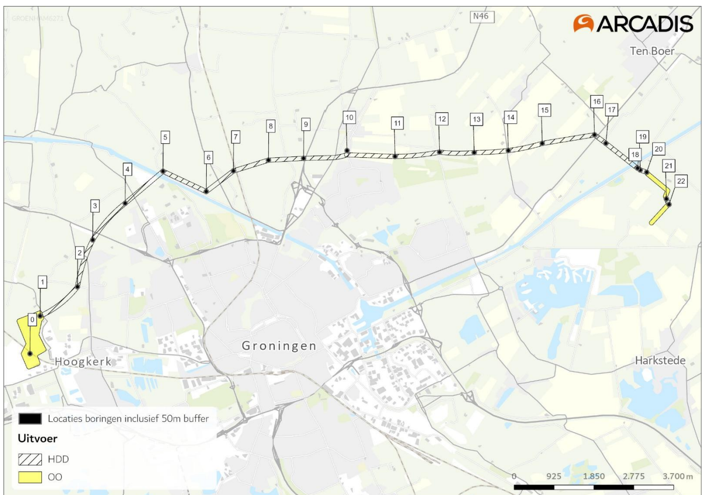
Figuur 5.8.4 Kabelverbinding met de boorpunten genummerd
