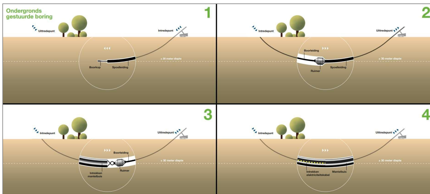
Figuur 2.4 Lengtedoorsnijing HDD boring
