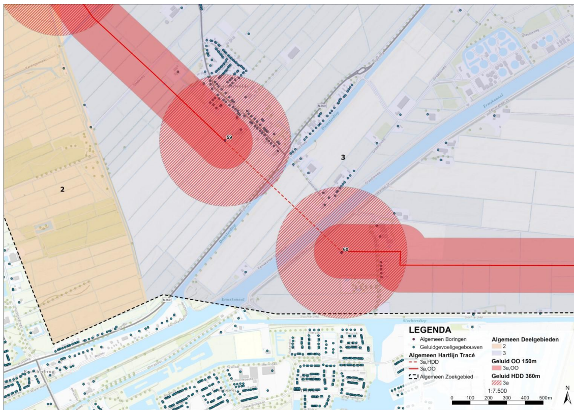
Figuur 8.13 Boring 59-60
