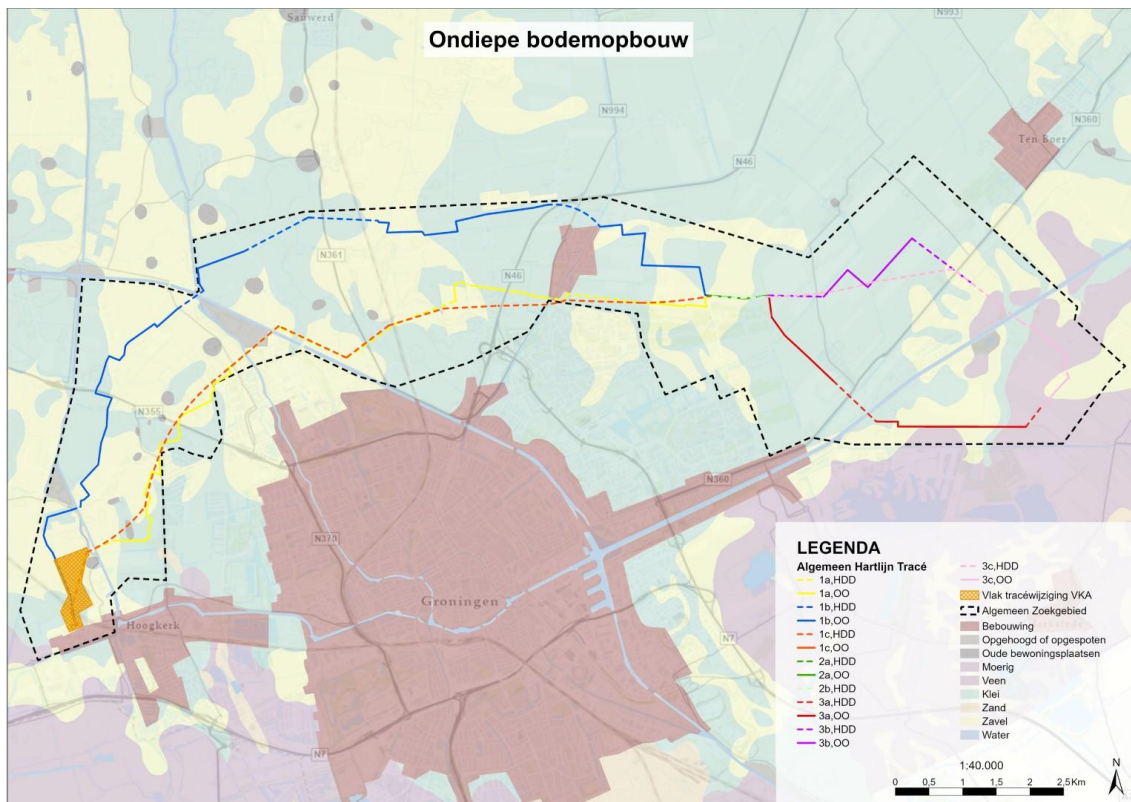
Figuur 3.3.2 Ondiepe bodemopbouw
