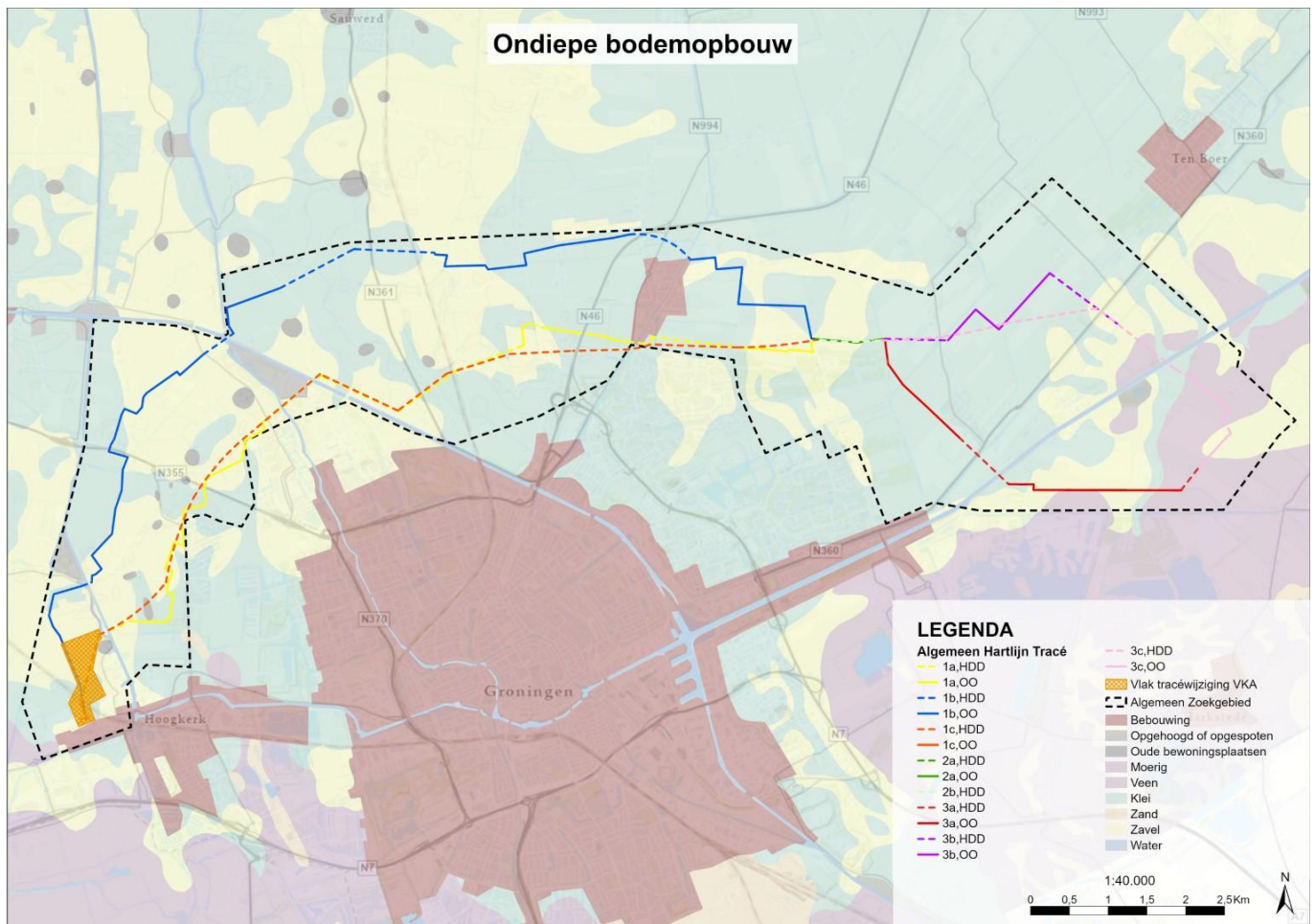
Figuur 4.3.2 Figuur 4.3.2 Ondiepe bodemopbouw
