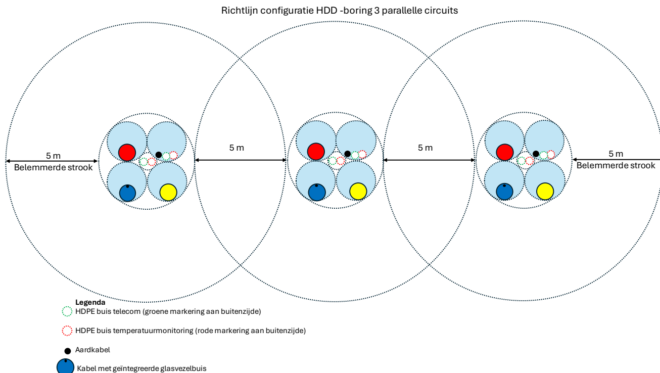
Figuur 2.3 Dwarsdoorsnede HDD boring (de rood, geel en blauwe bolletjes zijn de hoogspanningskabels)
