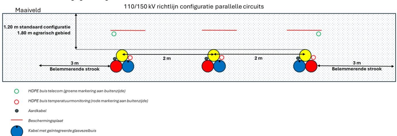
Figuur 2.1 Ligging in Open ontgraving (de rood, geel en blauwe bolletjes zijn de hoogspanningskabels)
