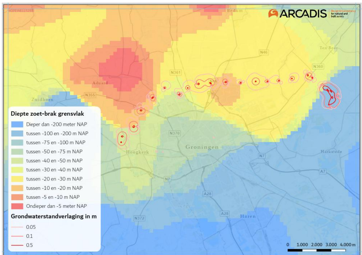
Figuur 4.8.2 Ligging brak en/of zout grondwater binnen de 0,05-m, 0,1-m en 0,5-m grondwaterstandverlaging invloedsgebieden van de bemalingen
