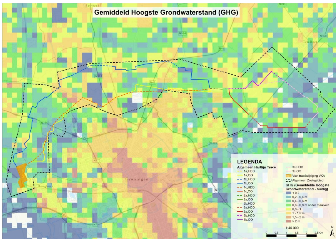
Figuur 3.3.3 Gemiddeld Hoogste Grondwaterstand (GHG)
