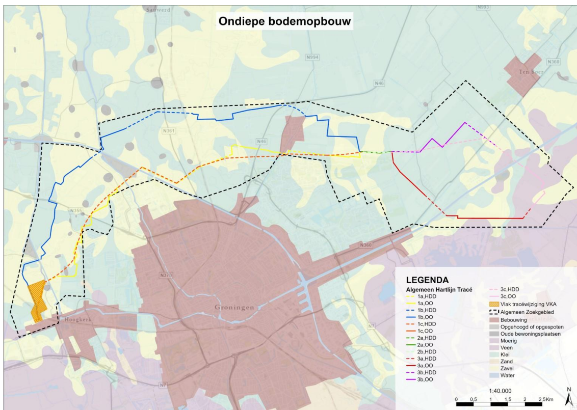
Figuur 3.3.1 Ondiepe bodemopbouw
