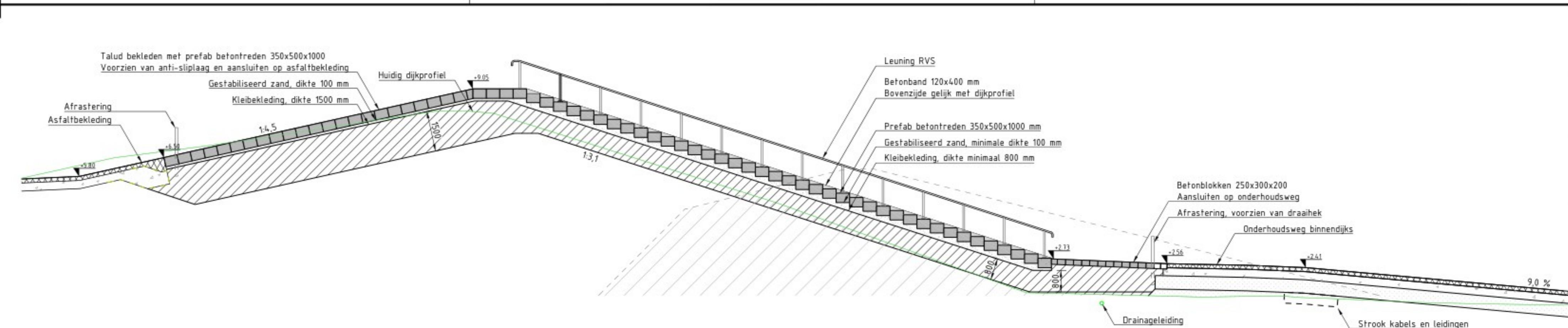
DOORSNEDE ONTWERP Schaal 1: 100
