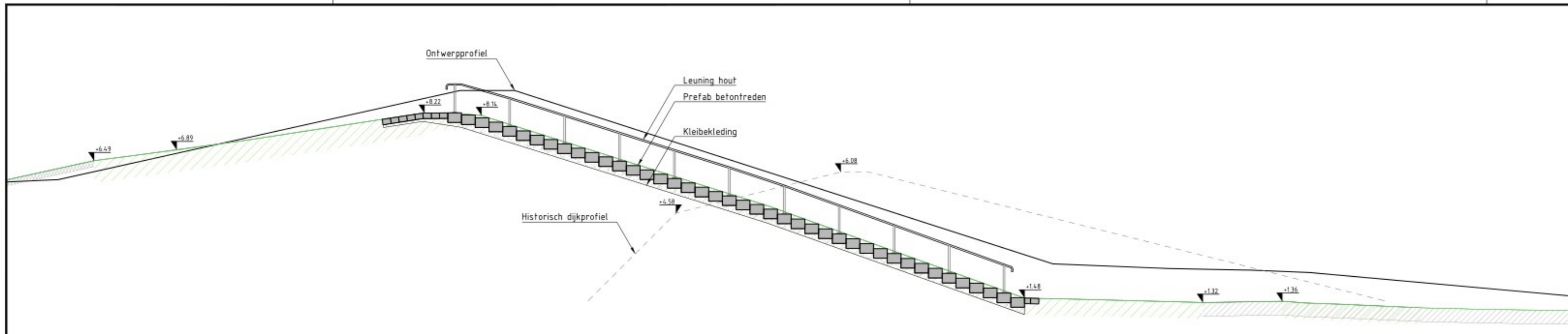
DOORSNEDE HUIDIGE SITUATIE Schaal 1: 100
