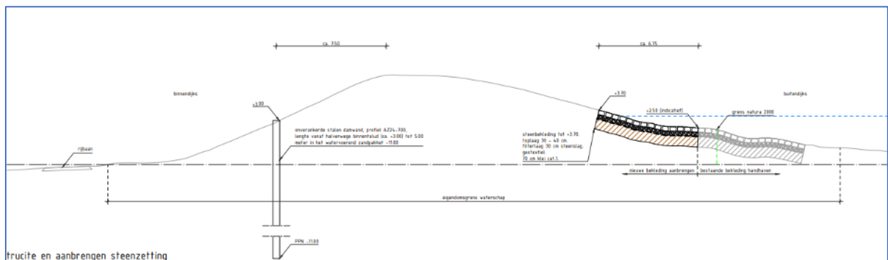
Figuur 0-3 Uitsnede uit het dwarsprofiel met maatregelen uit KA1 in dijkvak 1.
