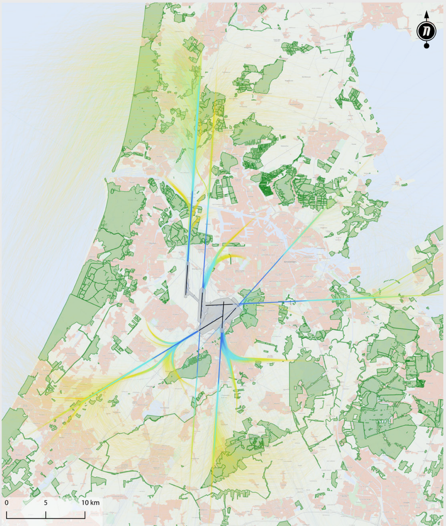
Figuur 15 - Vliegpaden en vlieghoogtes.
