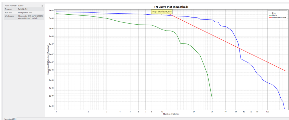
Figuur 8: Groepsrisico, FN-curven voor de dag- en nachtperiode inclusief kans op 10 slachtoffers (dagperiode)
