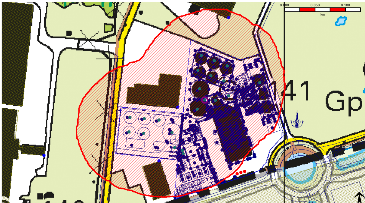
Figuur 7: Plaatsgebonden Risico-contouren (details)
