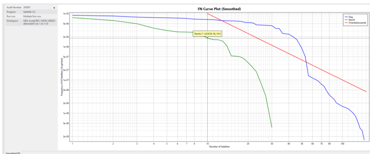
Figuur 9: Groepsrisico, FN-curven voor de dag- en nachtperiode inclusief kans op 10 slachtoffers (nachtperiode)
