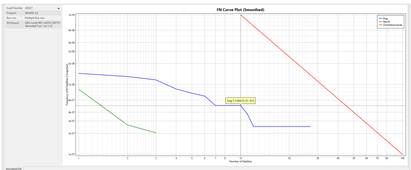
Figuur 12: Groepsrisico, FN-curven voor de dag- en nachtperiode inclusief kans op 10 slachtoffers (dagperiode)
