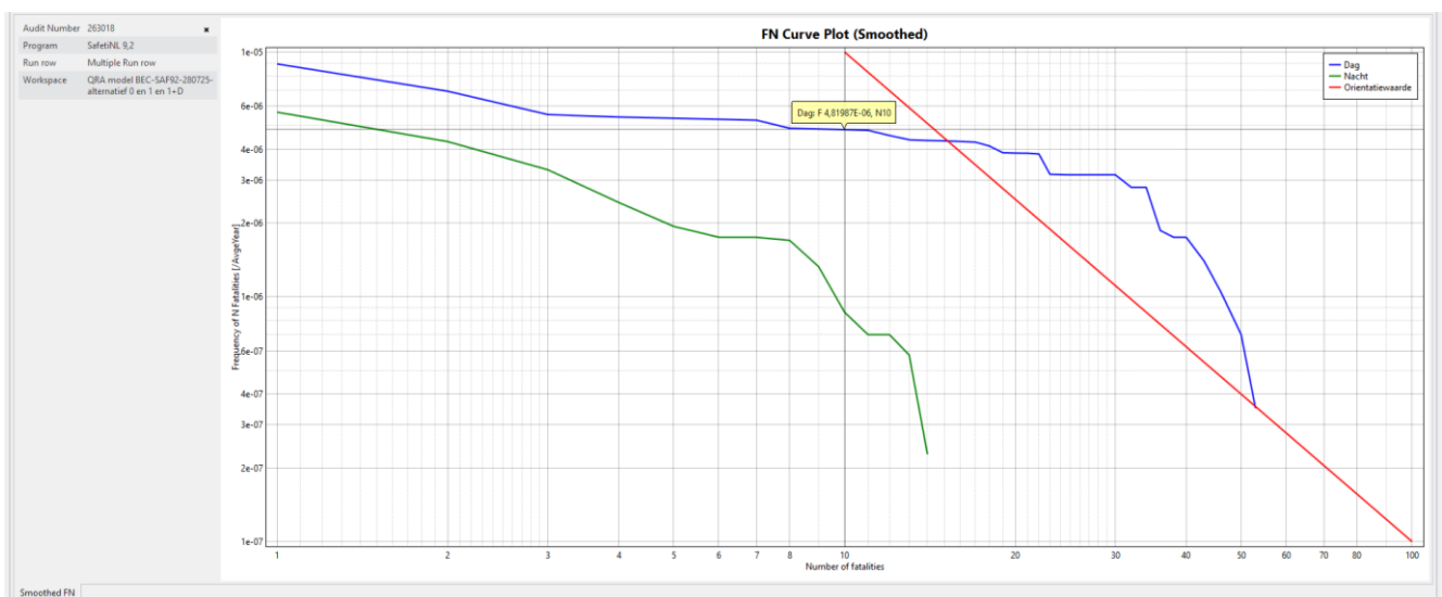
Figuur 4: Groepsrisico, FN-curve voor de dag- en nachtperiode inclusief kans op 10 slachtoffers (dagperiode)
