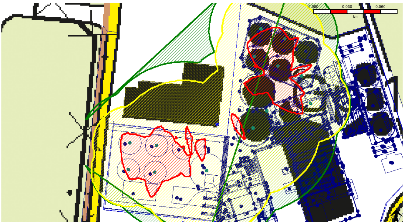
Figuur 11: Plaatsgebonden Risico-contouren (details) in het geval snelafsluiters worden toegepast
