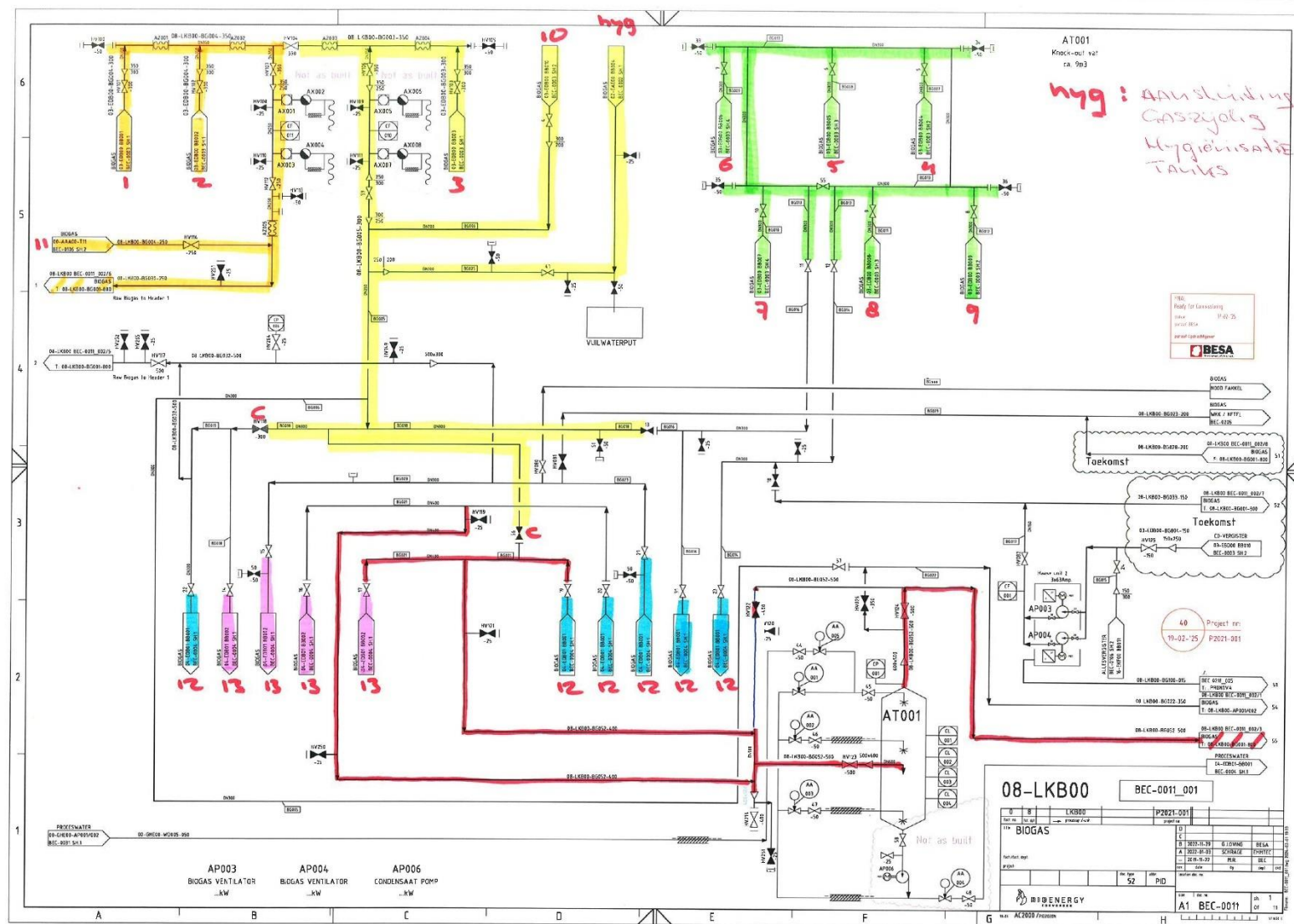
Bijlage-11: P&ID's met daarbij de posities van de afsluiters
