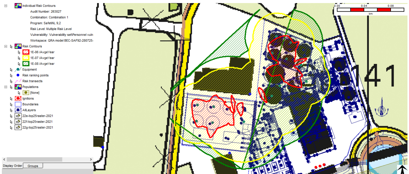
Figuur 10: Plaatsgebonden Risico-contouren in het geval snelafsluiters worden toegepast
