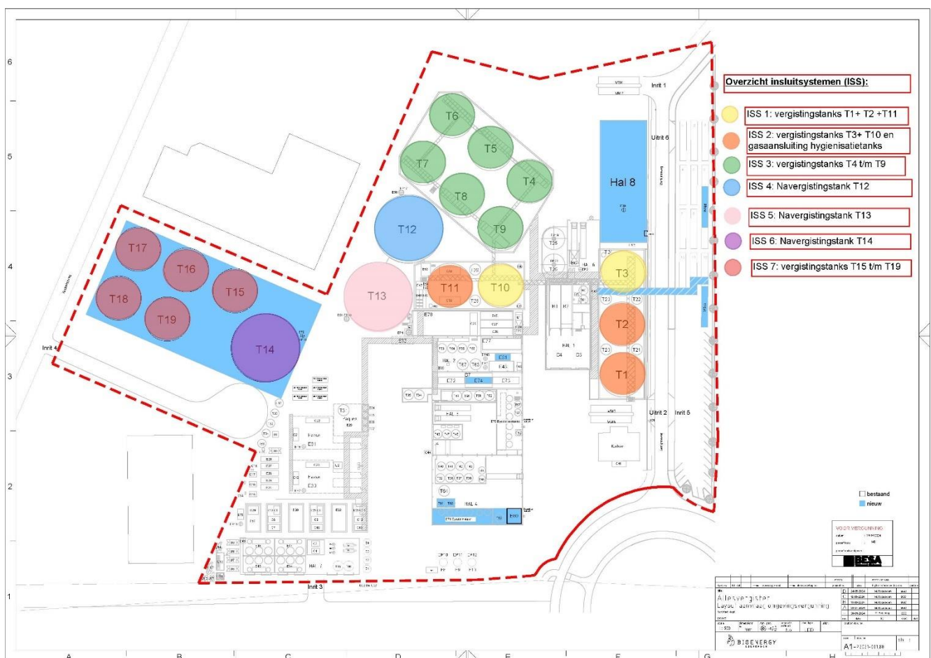
Figuur 9: Insluitsystemen na plaatsing snelafsluiters
