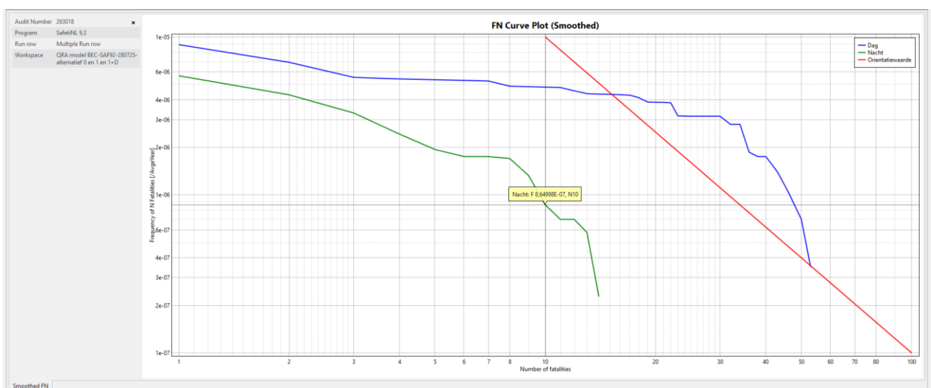
Figuur 5: Groepsrisico, FN-curve voor de dag- en nachtperiode inclusief kans op 10 slachtoffers (nachtperiode)
