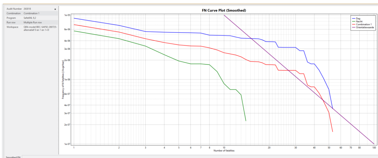
Figuur 6: Groepsrisico, FN-curves voor dag en nacht en gecombineerde FN-curve
