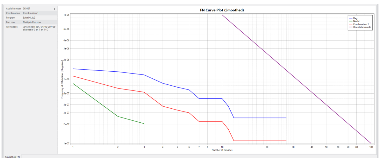
Figuur 13: Groepsrisico, FN-curves voor dag en nacht en gecombineerde FN-curve
