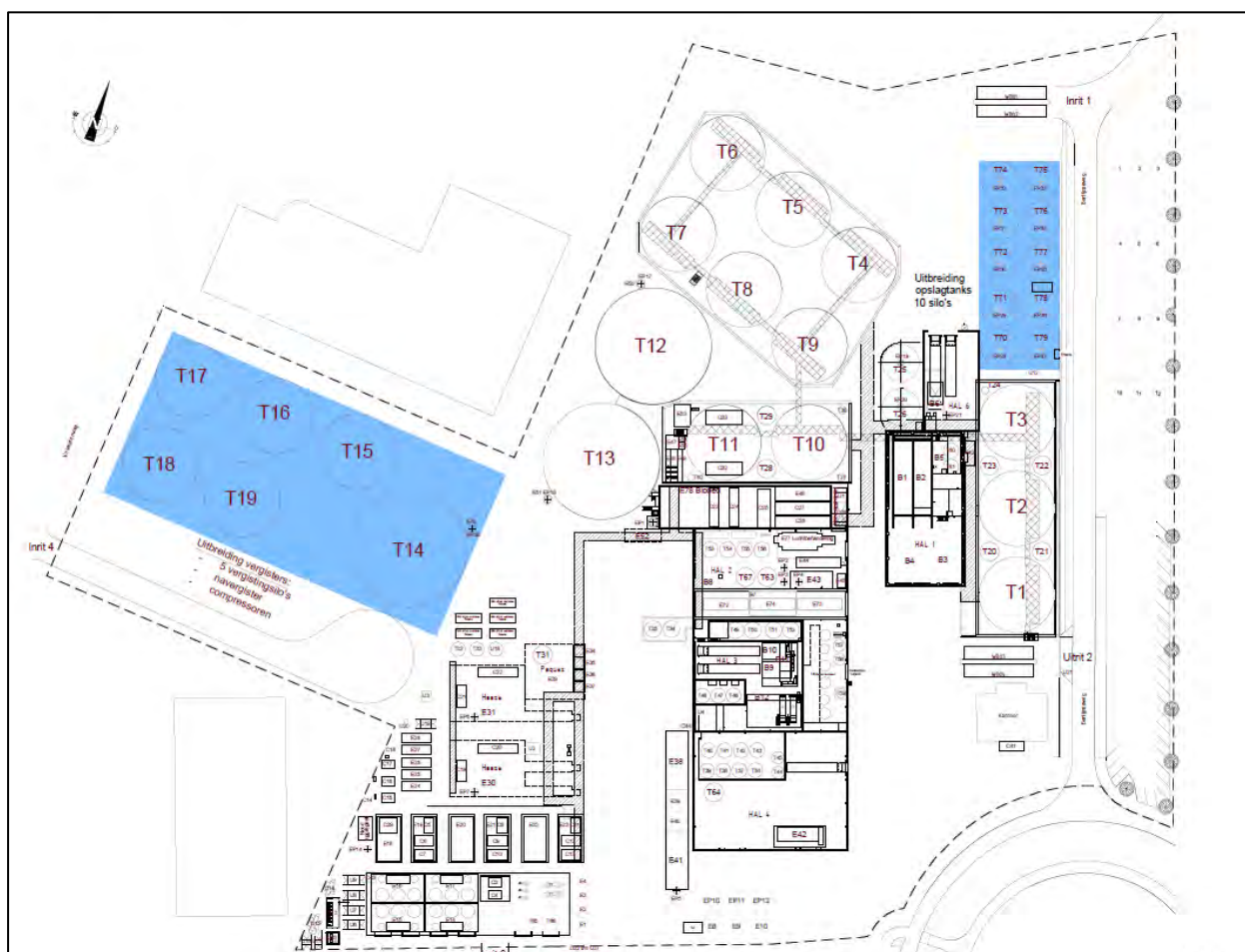
Figuur 2-b: Overzicht bedrijfsterrein voorgenomen activiteit (alternatief 1).
