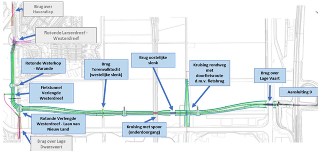
Afbeelding 6.2 Voorontwerp Rondweg Lelystad-Zuid*
