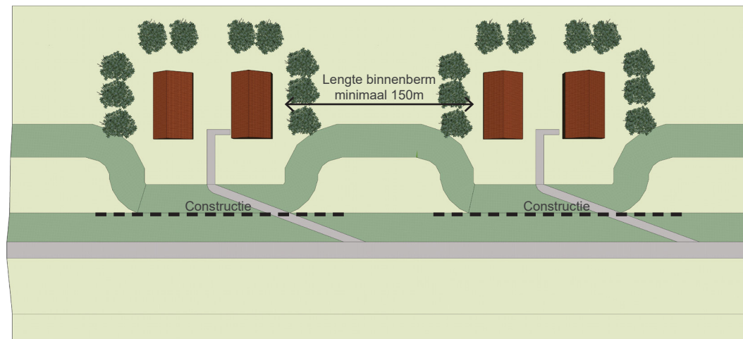
Figuur 59: onderbreking binnenbermen tussen individuele bebouwing met erven.
