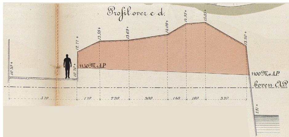
Figuur 66: profiel oude vesting ter hoogte van de Oliestraat (links weergegeven in het profiel) in Grave.
