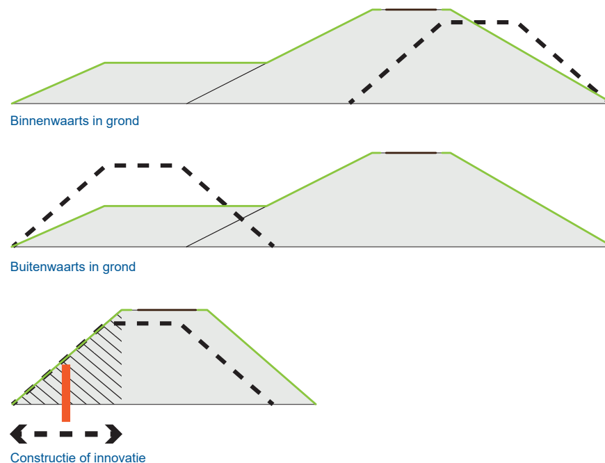
Figuur 24: hiërarchie voor versterking van de gronddijk.
