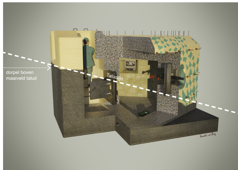
Figuur 61: impressie S3 Kazemat in het talud van de dijk.
