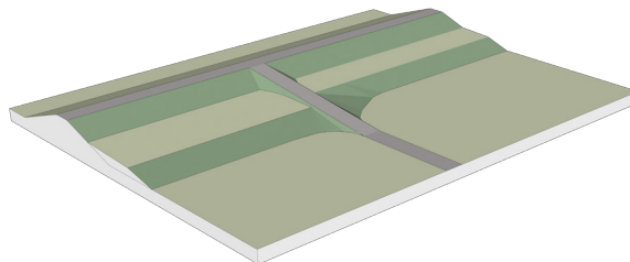
Figuur 35: overgang tussen binnenbermen van verschillende breedte.
