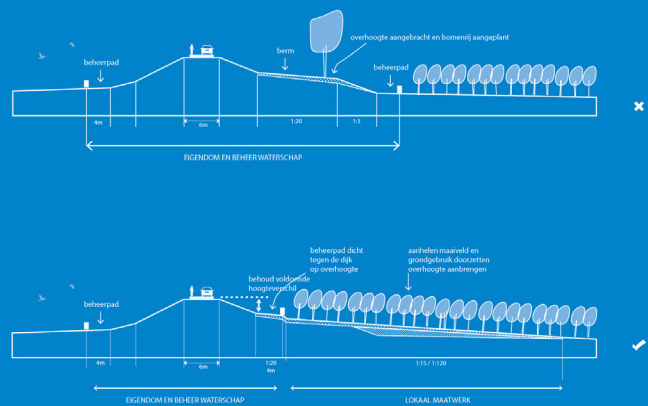
Figuur 8: inpassingsmaatregelen per faalmechanisme (bron: Ruimtelijk Kwaliteitskader Cuijk-Ravenstein).
