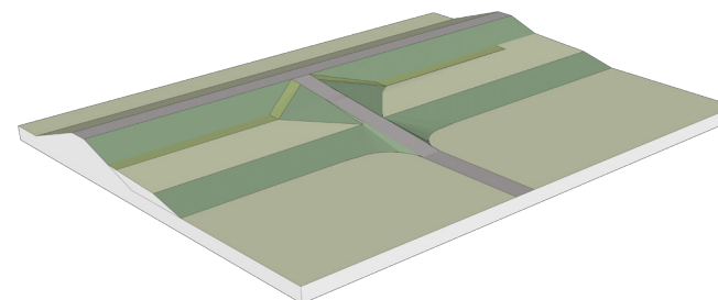
Figuur 43: toegang naar beheerstrook via de oksel van de oprit.
