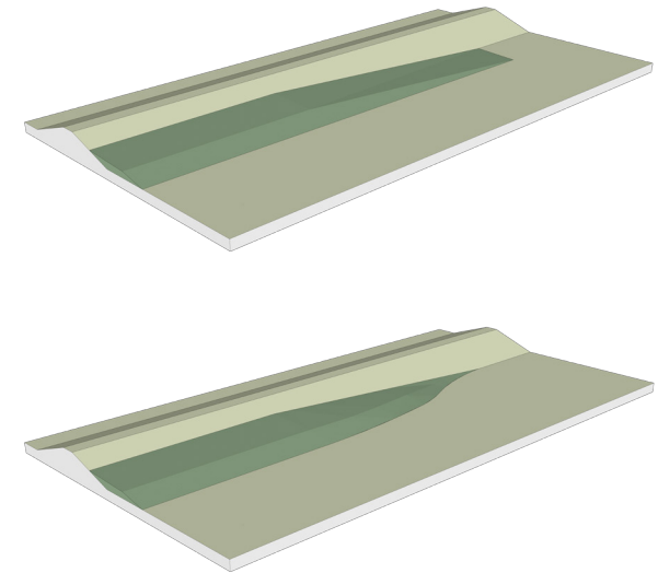
Figuur 33: vloeiend vormgegeven overgangen tussen dijkprofielen.
