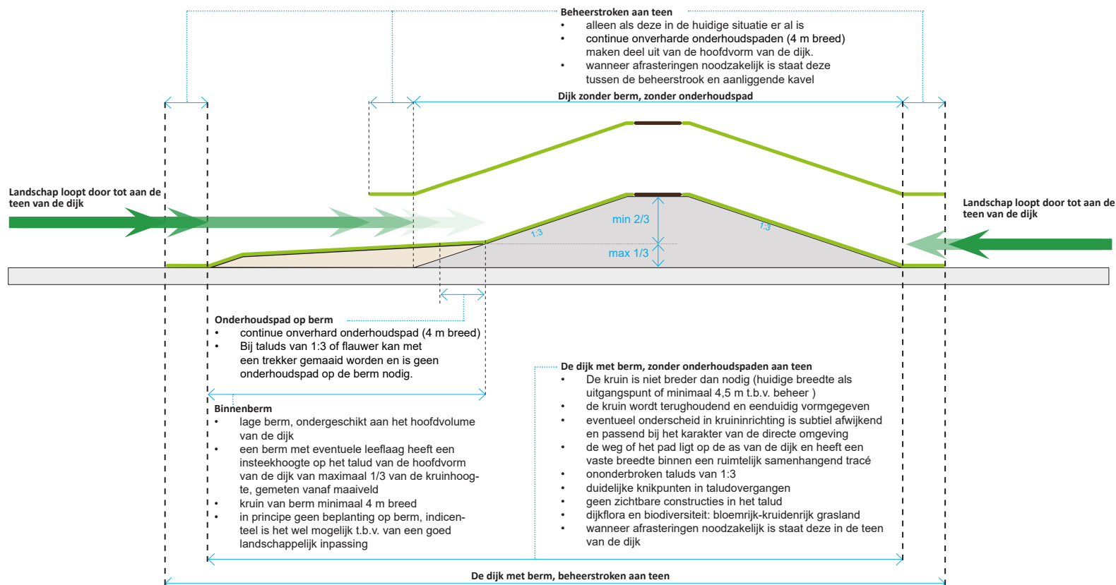
Figuur 26: principeprofiel dijk
