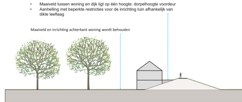
Figuur 46: inpassing dijkhuizen op de dijk.
