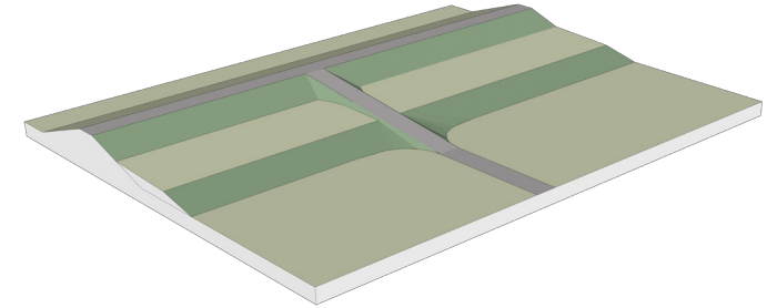
Figuur 41: oprit naar van aansluitende weg, haaks op de dijk.
