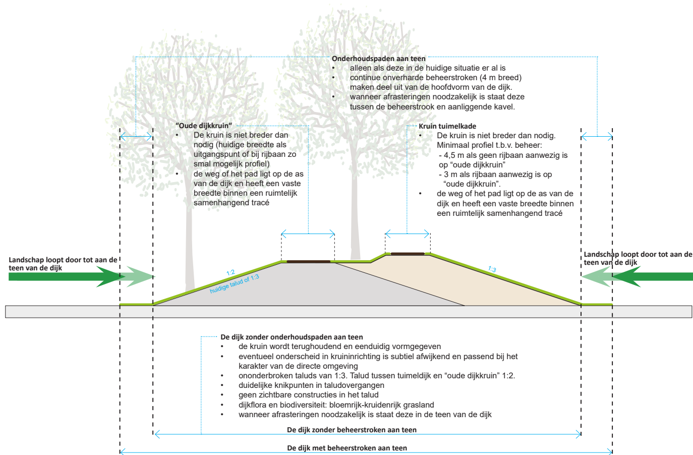
Figuur 28: principeprofiel dijk met tuimelkade.
