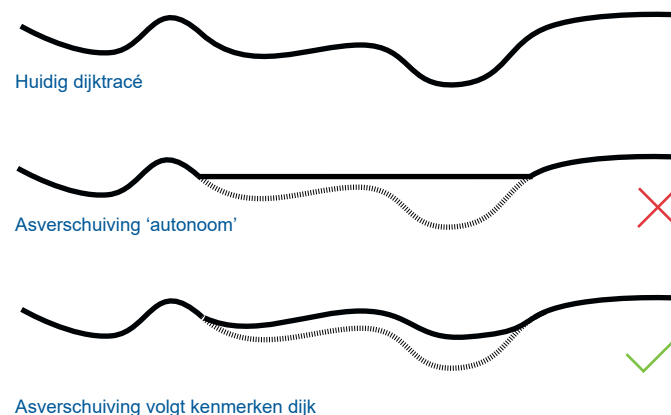
Figuur 31: huidige tracé is het uitgangspunt.
