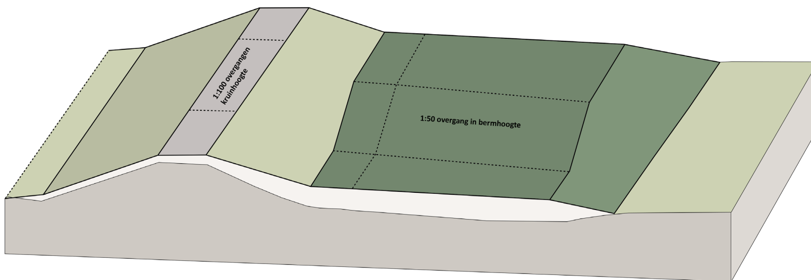
Figuur 38: schematische weergave van overgangen in kruinhoogtes en bermhoogtes.
