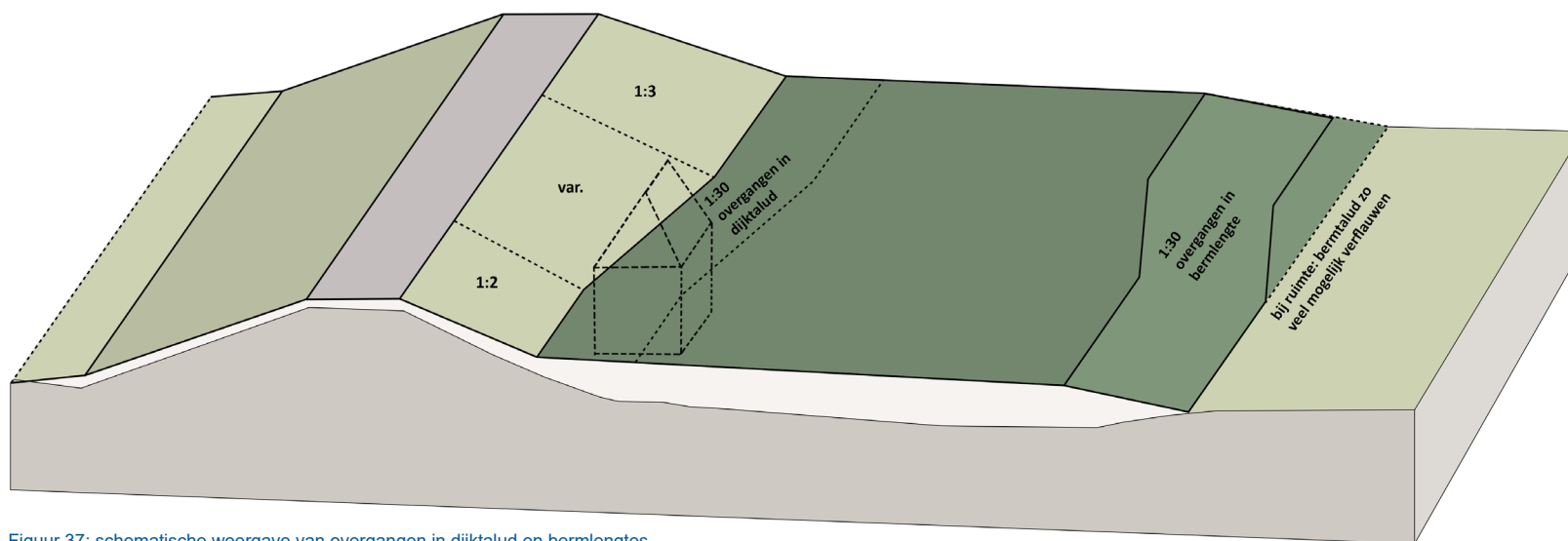
Figuur 37: schematische weergave van overgangen in dijkwalud en bermhoogtes.
