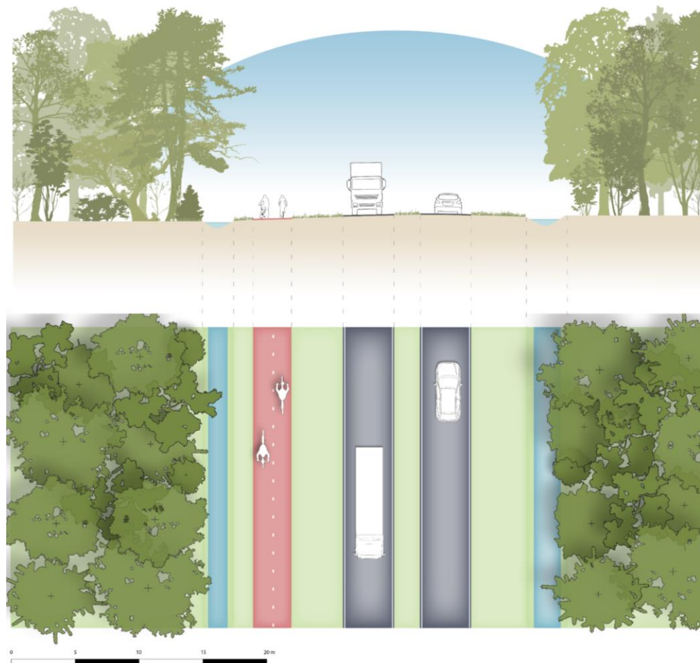
Figuur 34 Dwarsprofiel Zandbos richting Deurne in gebied B
