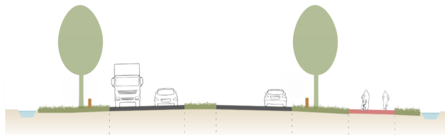
Figuur 26 Opzet wegprofiel met krappe obstakelvrije ruimte; behoud bomen naast de rijbanen met geleiderails.
