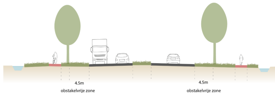
Figuur 25 Voorkeursprincipe: begeleidende bomenrijen langs de rijbanen als schakel tussen weg en het omgevend landschap
