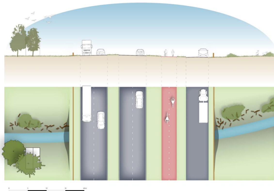
Figuur 33 boven: Dwarsprofiel Oude Aa in gebied A.
