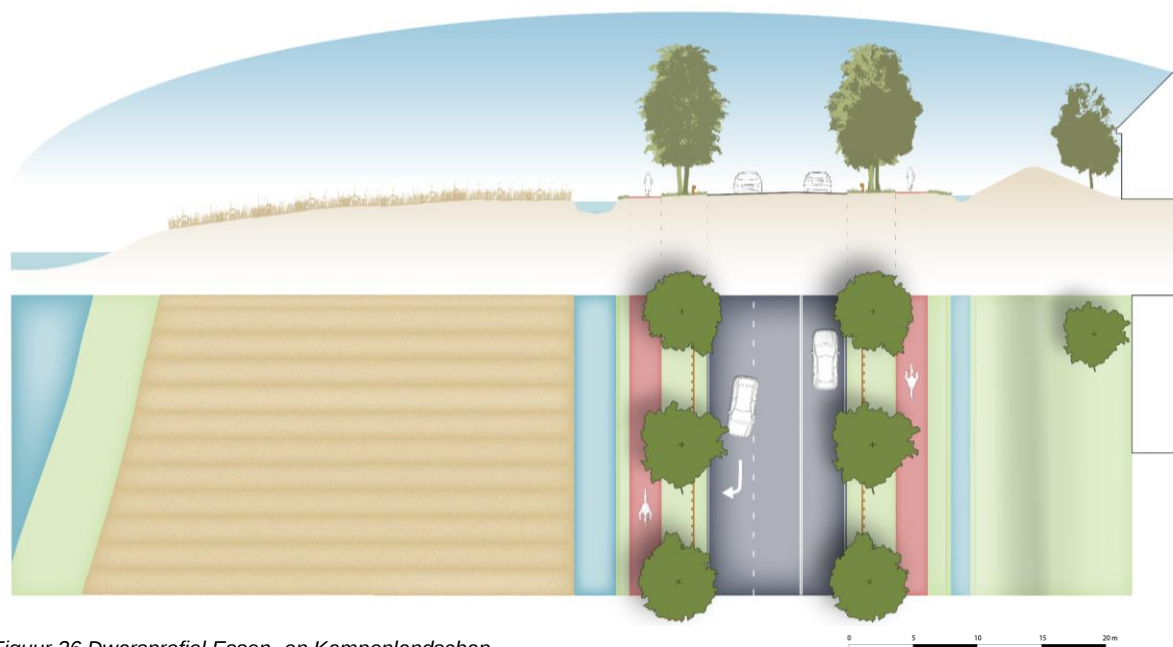
Figuur 36 Dwarsprofiel Essen- en Kampenlandschap
