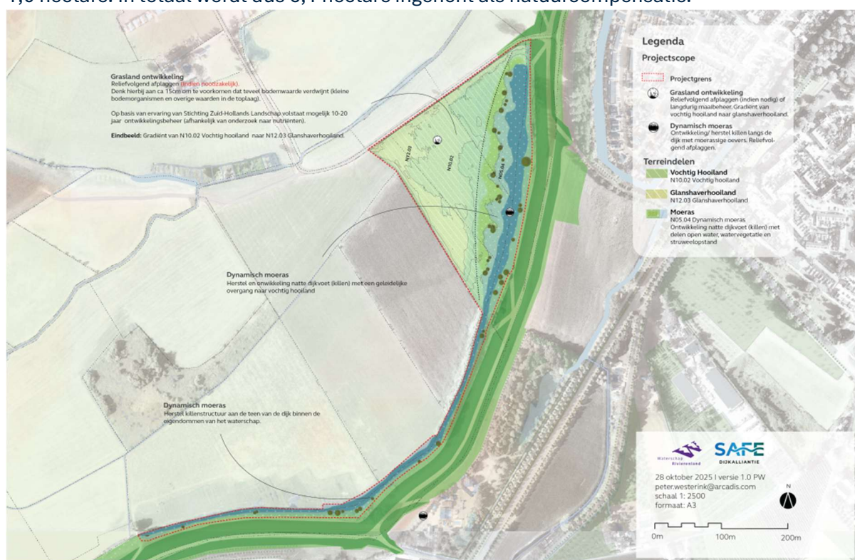
Figuur 2-1: vergunningenontwerp ter plaatse van compensatielocatie Polder de Eendracht
