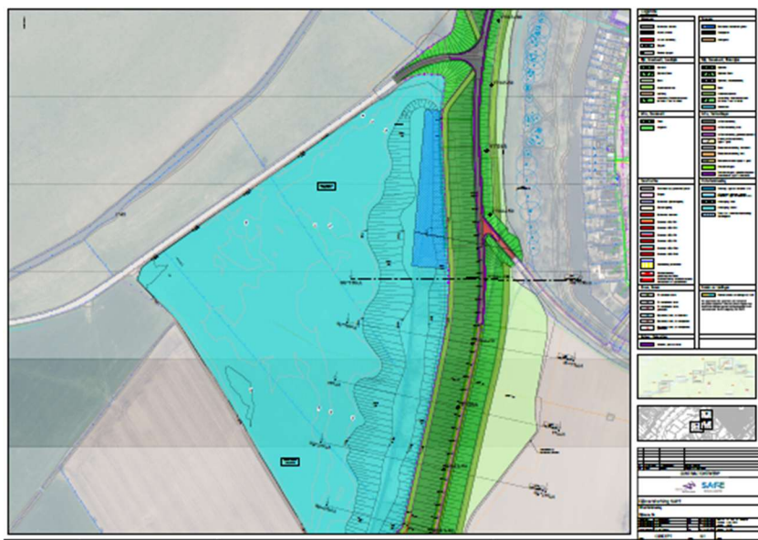
Figuur 2-2: contractontwerp Polder de Eendracht
