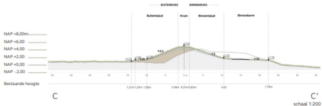
Figuur 2-18: Dwarsprofiel CC' met asverschuiving buitenwaarts.
