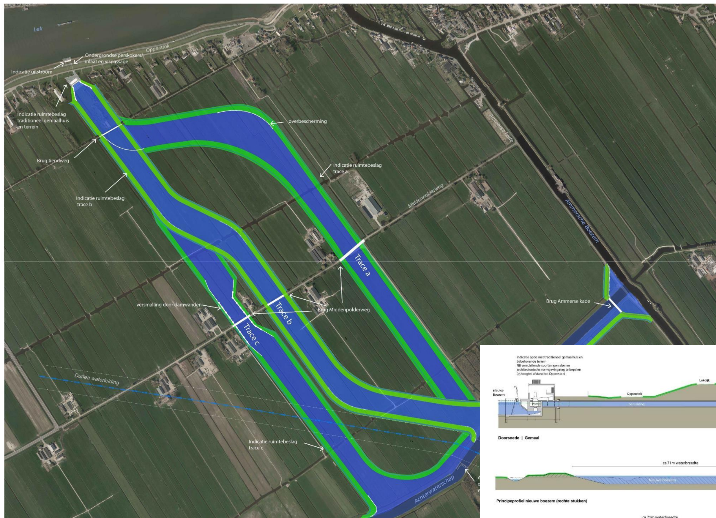
Figuur S5: Kaart met schetsontwerp boezem en gemaal Groot-Amers West incl. dwarsdoorsnedes.
