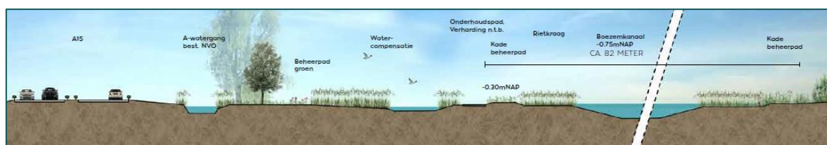
Figuur 5.9 Doorsnede van profiel 1: A-watergang, A15, watercompensatie en het boezemkanaal (bron: Van den Hurk, 2025).
