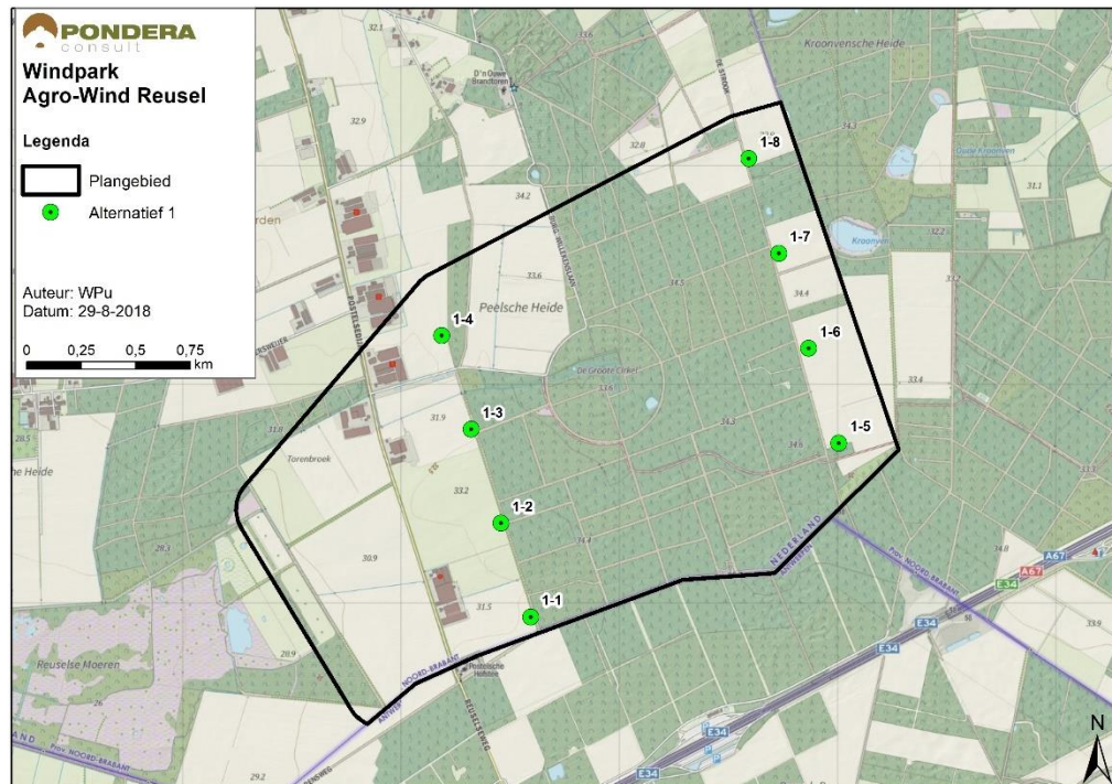
Figuur 1.6 Opstelling alternatief 1
