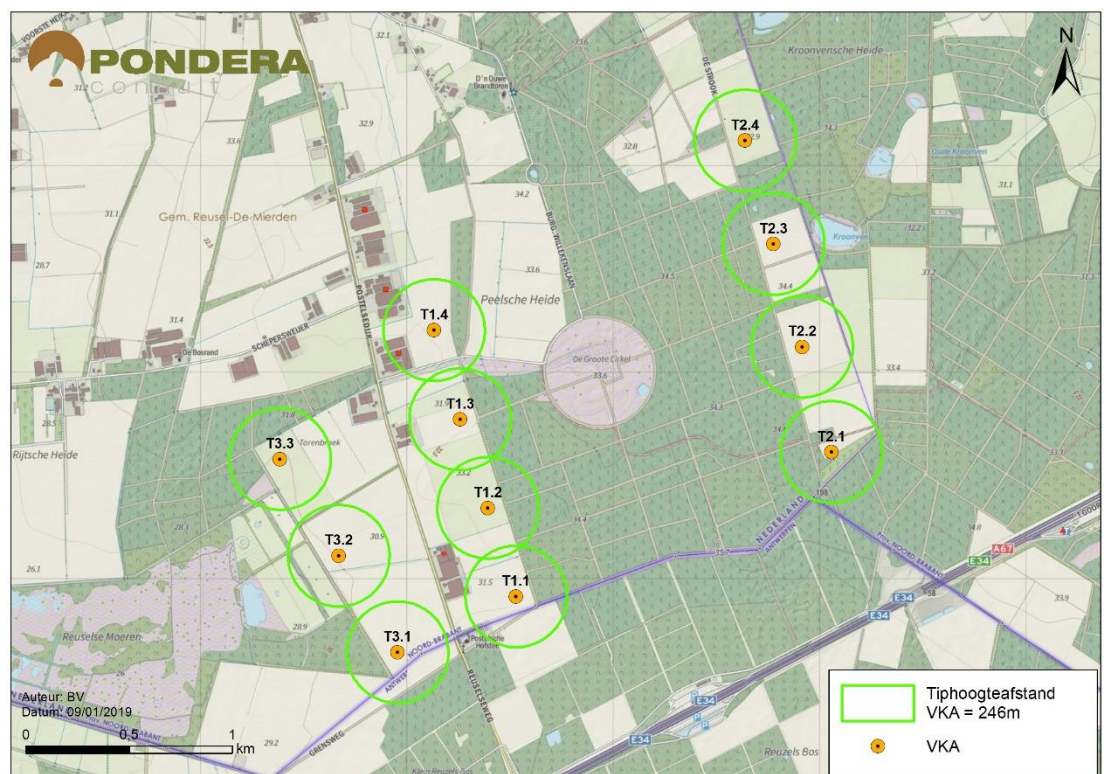
Figuur 17.11 Weergave maximale ligging PR10^{-06} contouren voorkeursalternatief
