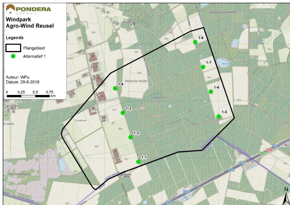
Figuur 4.1 Opstelling alternatief 1
