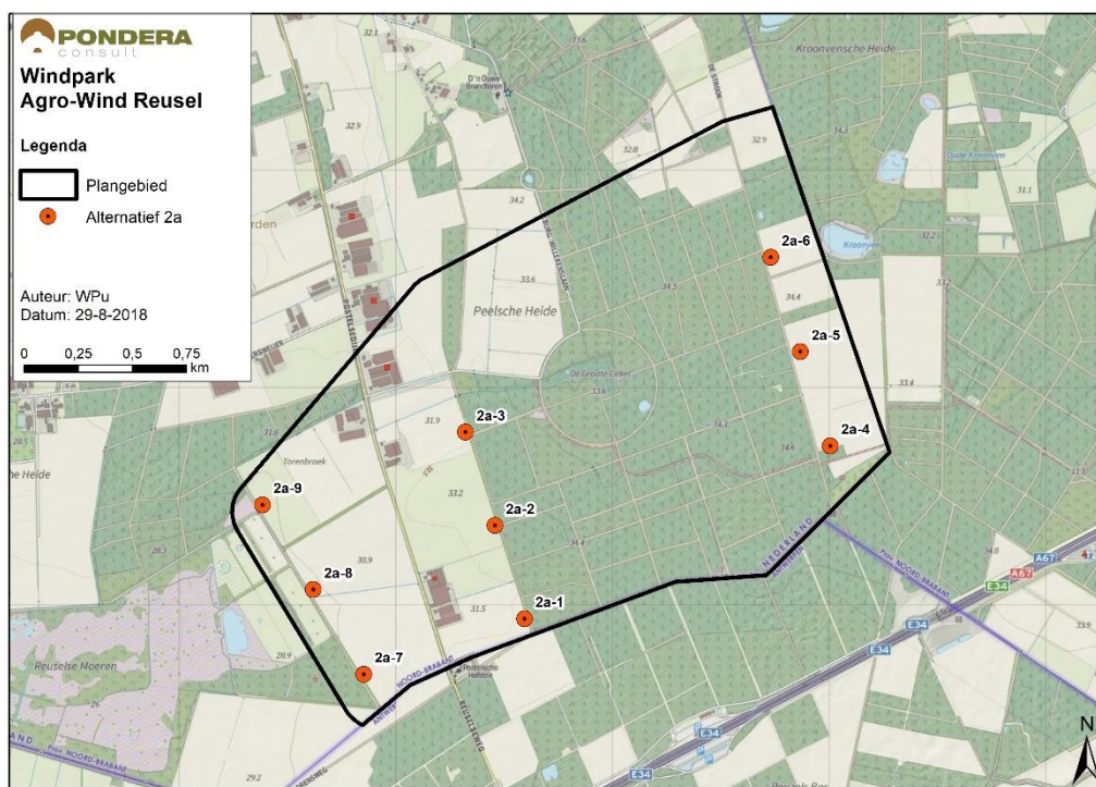
Figuur 1.7 Opstelling alternatief 2a
