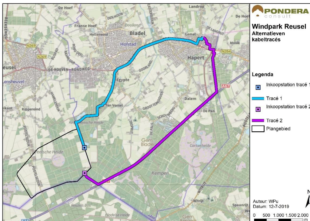
Figuur 9.10 Kabeltracé-alternatieven
