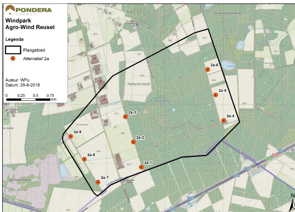
Figuur 4.2 Opstelling alternatief 2a
