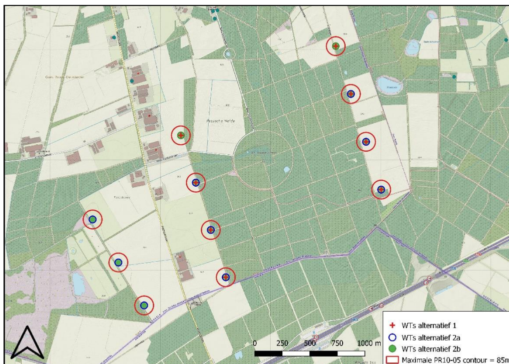
Figuur 12.2 Weergave maximale ligging PR10^{-05} contour alle opstellingsvarianten
