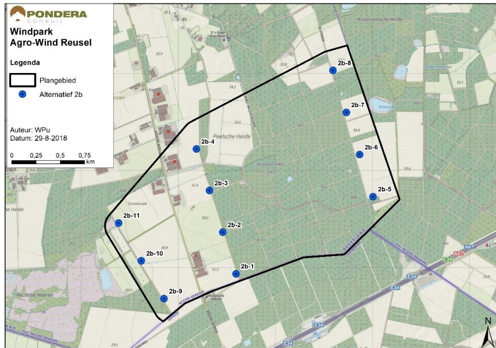
Figuur 4.3 Opstelling alternatief 2b
