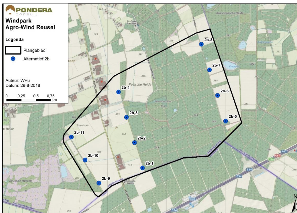
Figuur 1.8 Opstelling alternatief 2b
