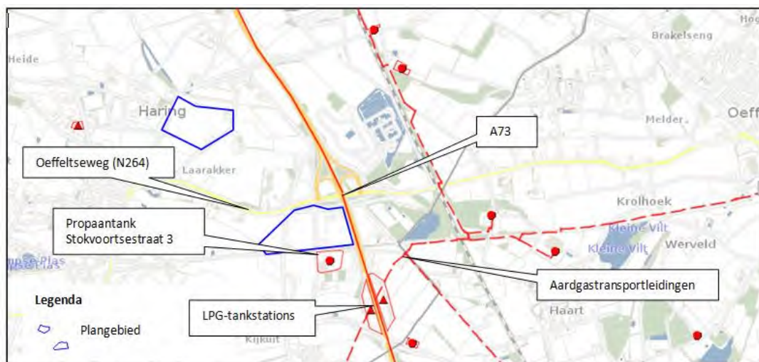
figuur 8.1 Risicobronnen omgeving plangebied
