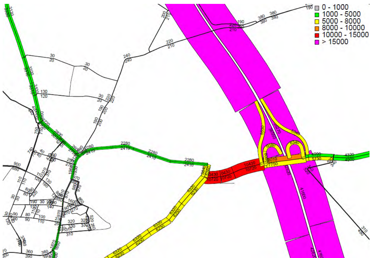
figuur 5.8 Verkeersintensiteiten (werkdag) in de referentiesituatie 2025
