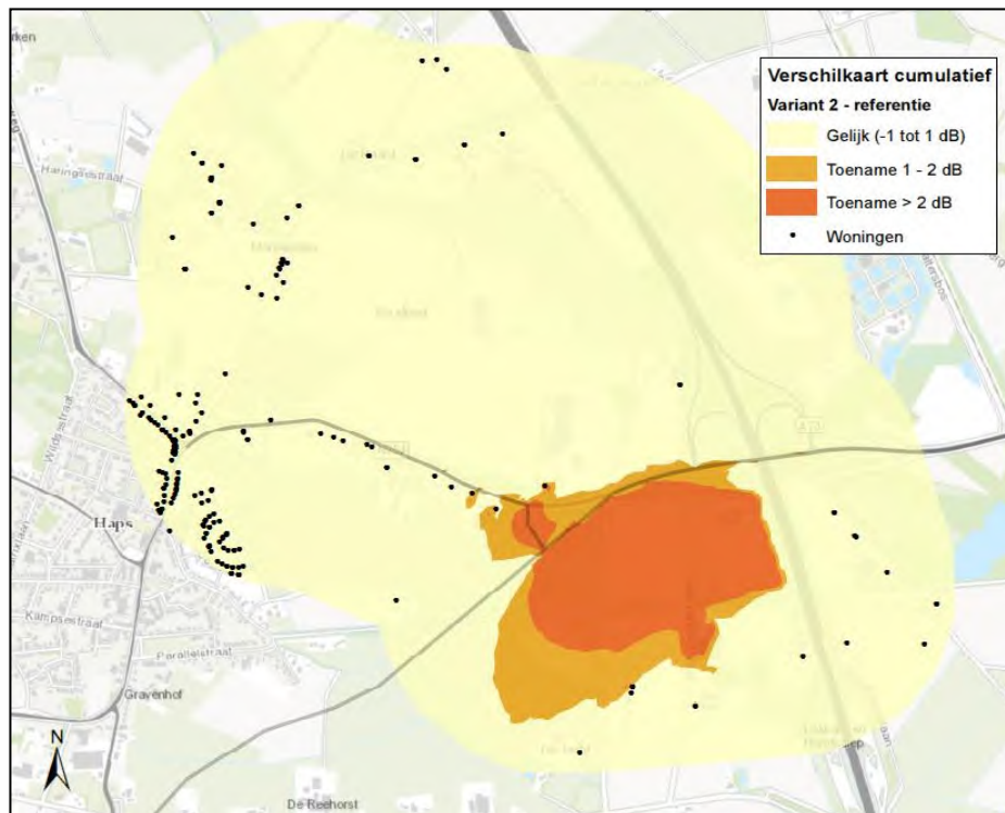
figuur 6.9 Verschilkaart gecumuleerde geluidbelasting L_{etm} industrie + wegverkeer variant 2 2025
