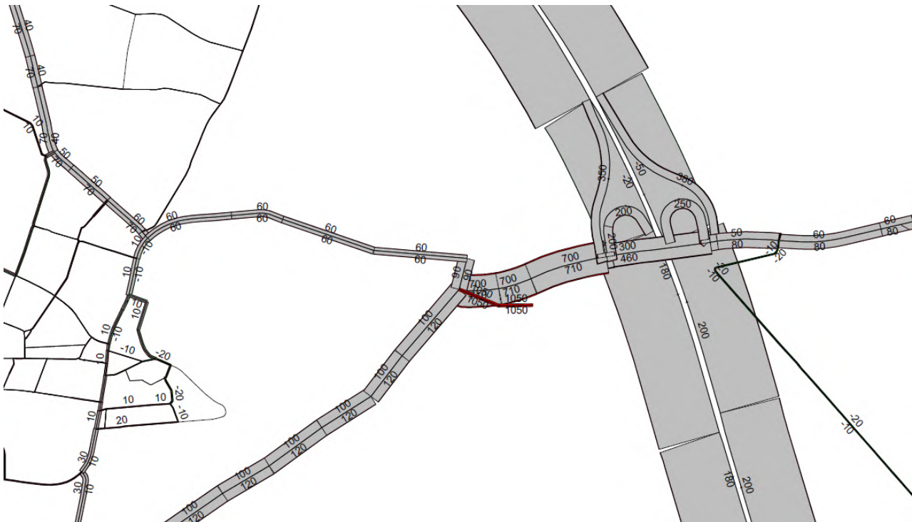
figuur 5.11 Toename verkeer (mvt/etmaal: werkdag) plansituatie (variant 1 en 2) versus de referentiesituatie
