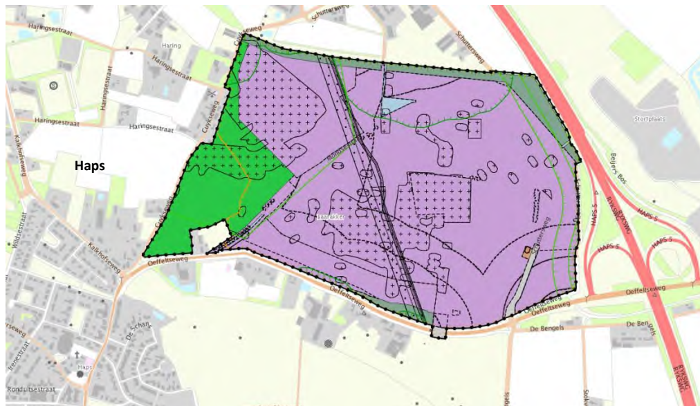
figuur 4.1 Plangebied Bedrijvenpark Laarakker conform het bestemmingsplan Bedrijvenpark Laarakker (Croonen, 2009)
