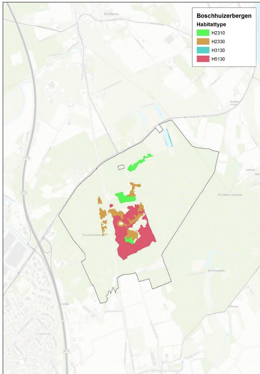
figuur 5.14. Habitattypenkaart Boschhuizerbergen met de habitattypen Stuifzandheiden (H2310), Zandverstuivingen (H2330), Zwakgebufferde vennen (H3130), Jeneverbesstruwelen (H5130).
