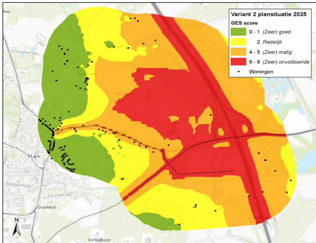
figuur 10.3 Gecumuleerde geluidbelasting GES plansituatie 2025 variant 2
