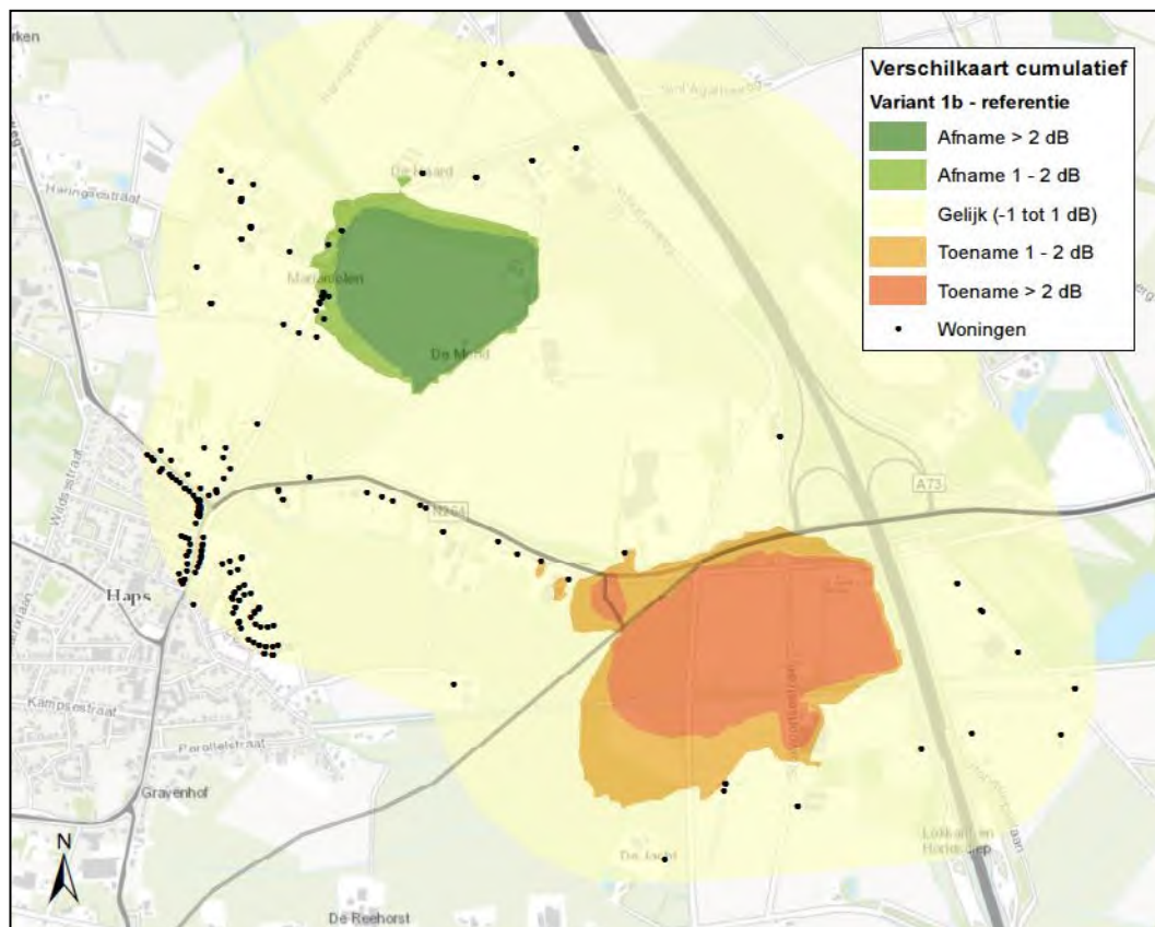
figuur 15.3 Verschilcontouren geluidbelasting L_{etm} gecumuleerd variant Tijdelijke uitruil (ten opzichte van de referentiesituatie)
