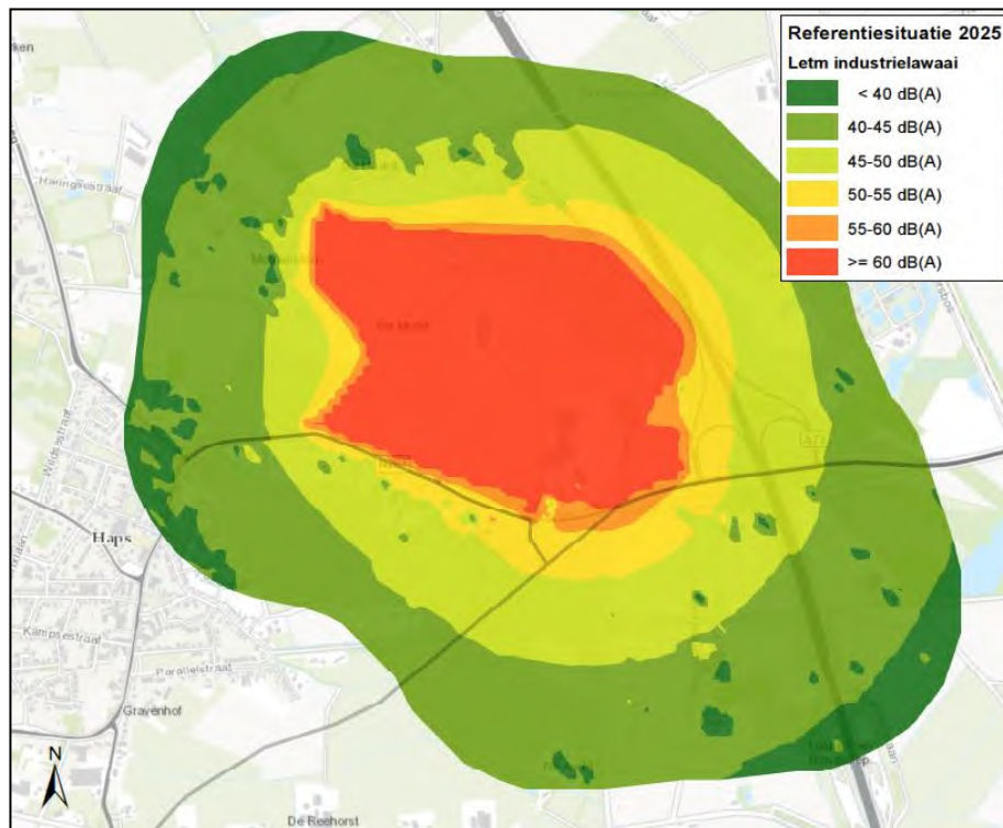
figuur 6.2 Geluidcontouren geluidbelasting L_{etm} industrie referentiesituatie 2025
