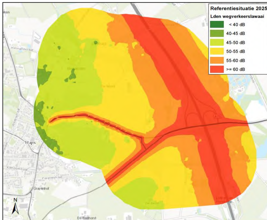
figuur 6.3 Geluidcontouren geluidbelasting L_{den} wegverkeer referentiesituatie 2025
