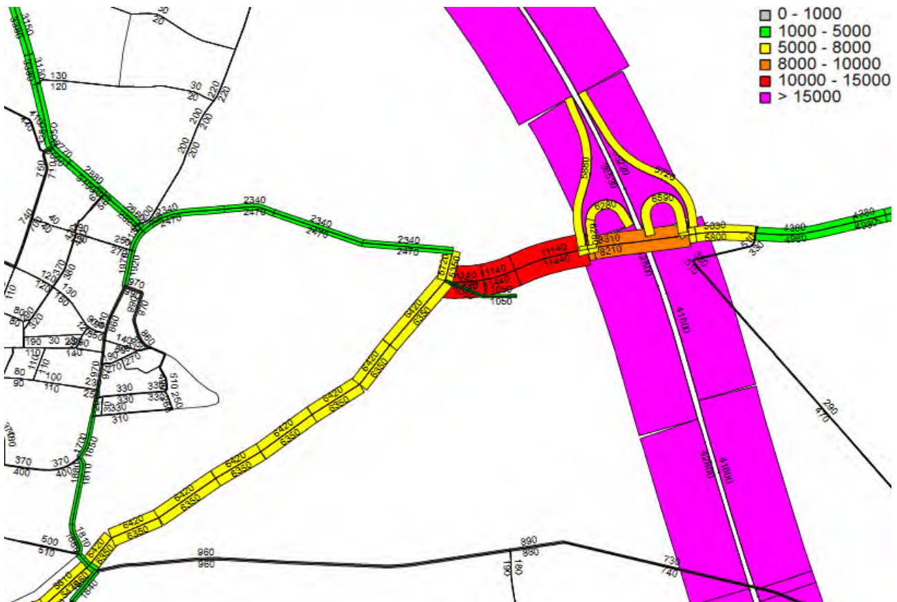
figuur 15.2 Etmaalintensiteiten (werkdag) variant Tijdelijke uitruil
