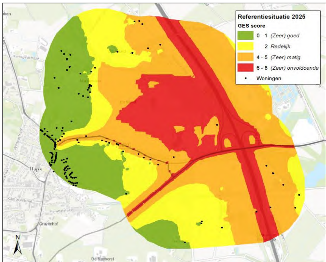
figuur 10.1 Gecumuleerde geluidbelasting in GES-scores voor de referentiesituatie
