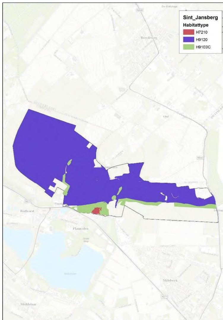
figuur 5.5 Habitattypenkaart Natura 2000-gebied Sint Jansberg met de habitattypen Galigaan-moerassen (H7210), Beuken-eikenbossen met hulst (H9120) en Vochtige alluviale bossen (H91E0C).
