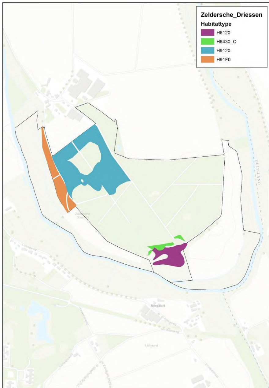
figuur 5.9 Habitattypenkaart Zeldersche Driessen met de habitattypen Stroomdalgraslanden (H6210), Ruigten en zomen (H6430C), Beuken-eikenbossen met hult (H9210) en Droge hardhoutooibossen (H91F0).
