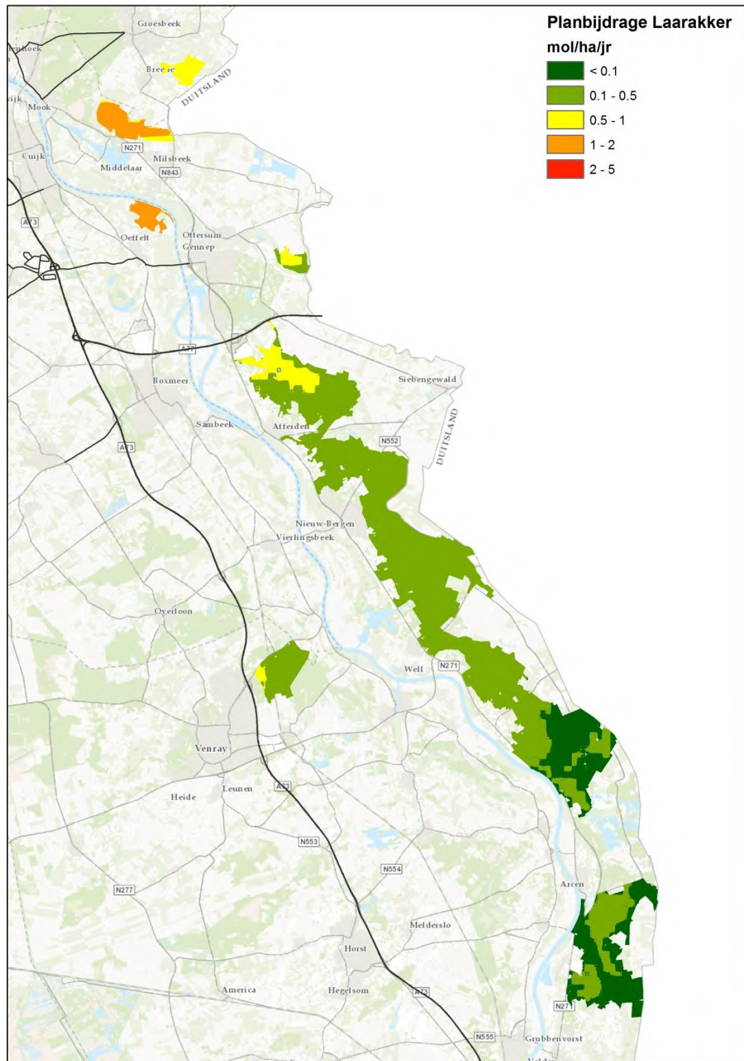
figuur 13.4 Stikstofdepositie op de aanwezige Natura 2000-gebieden
