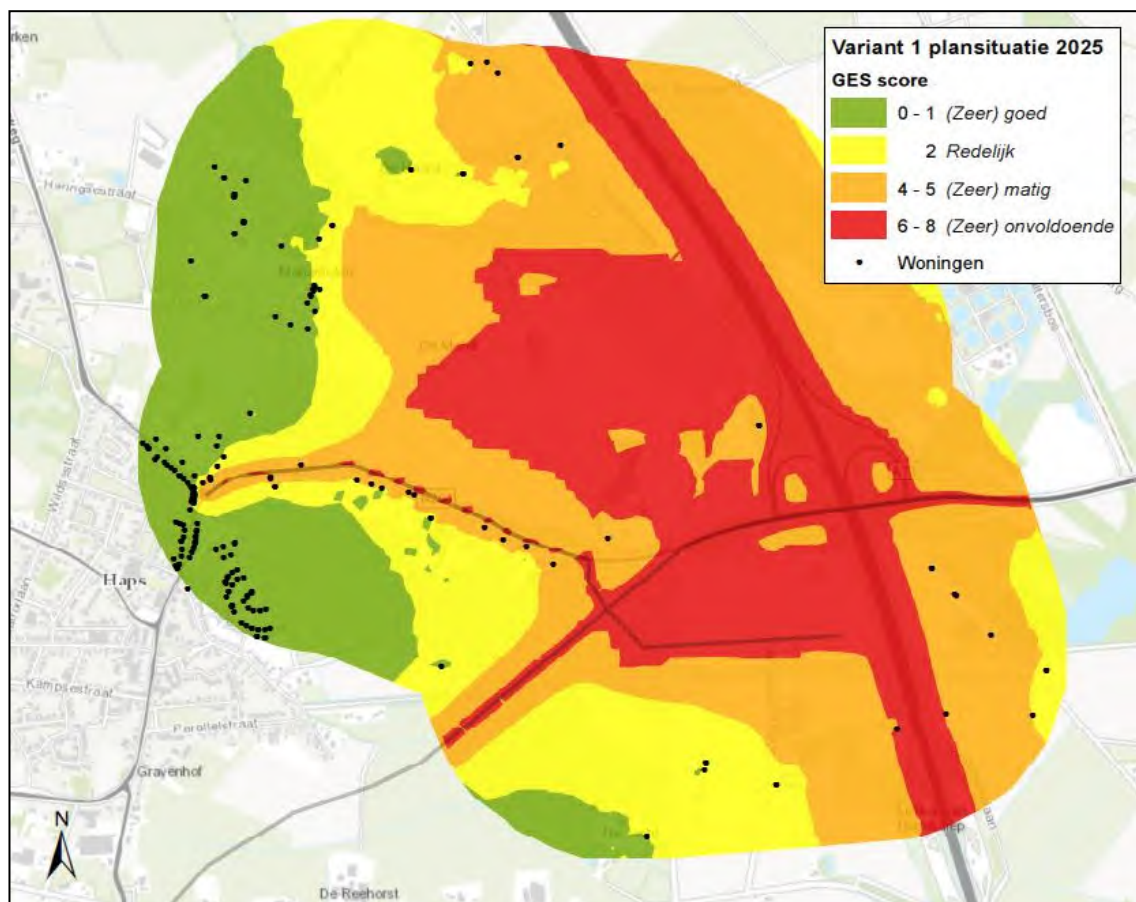
figuur 10.2 Gecumuleerde geluidbelasting GES plansituatie 2025 variant 1
