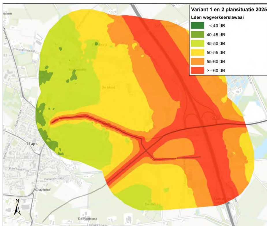
figuur 6.6 Geluidcontouren geluidbelasting L_{den} wegverkeer plansituatie (variant 1 en 2) 2025
