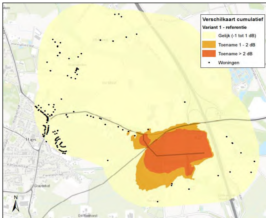
figuur 6.7 Verschilkaart gecumuleerde geluidbelasting L_{etm} industrie + wegverkeer variante 1 2025
