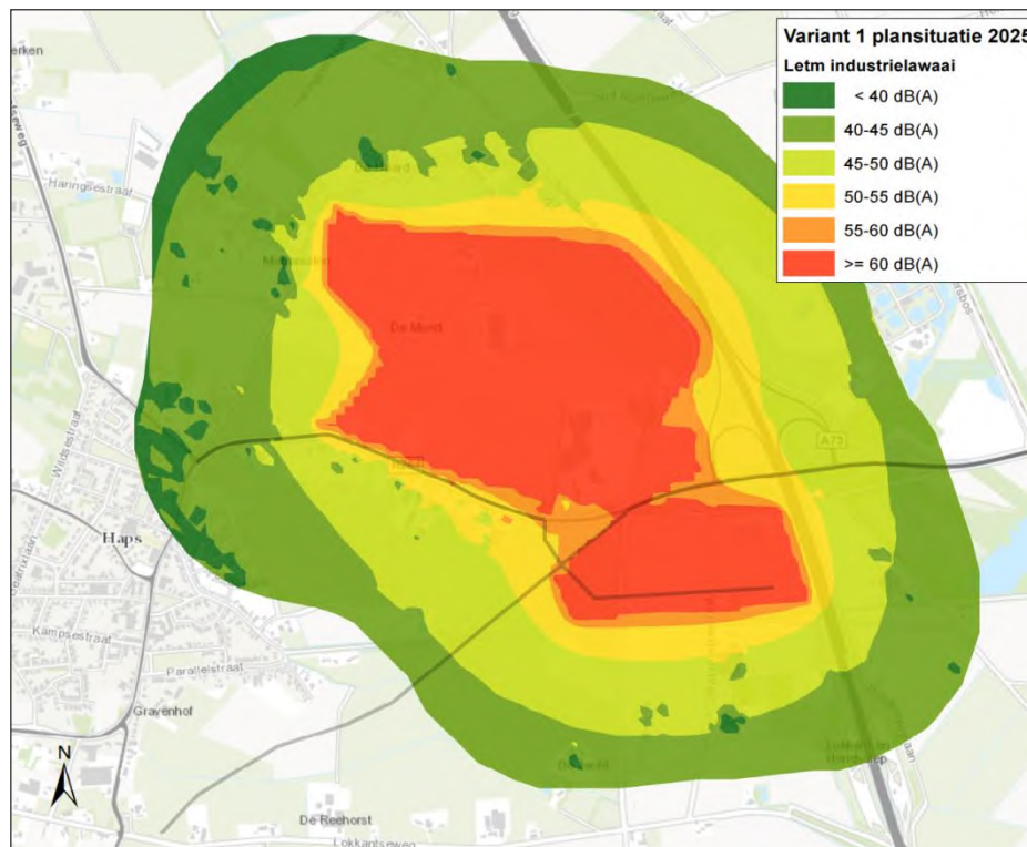
figuur 6.4 Geluidcontouren geluidbelasting L_{etm} industrie plansituatie variant 1 2025
