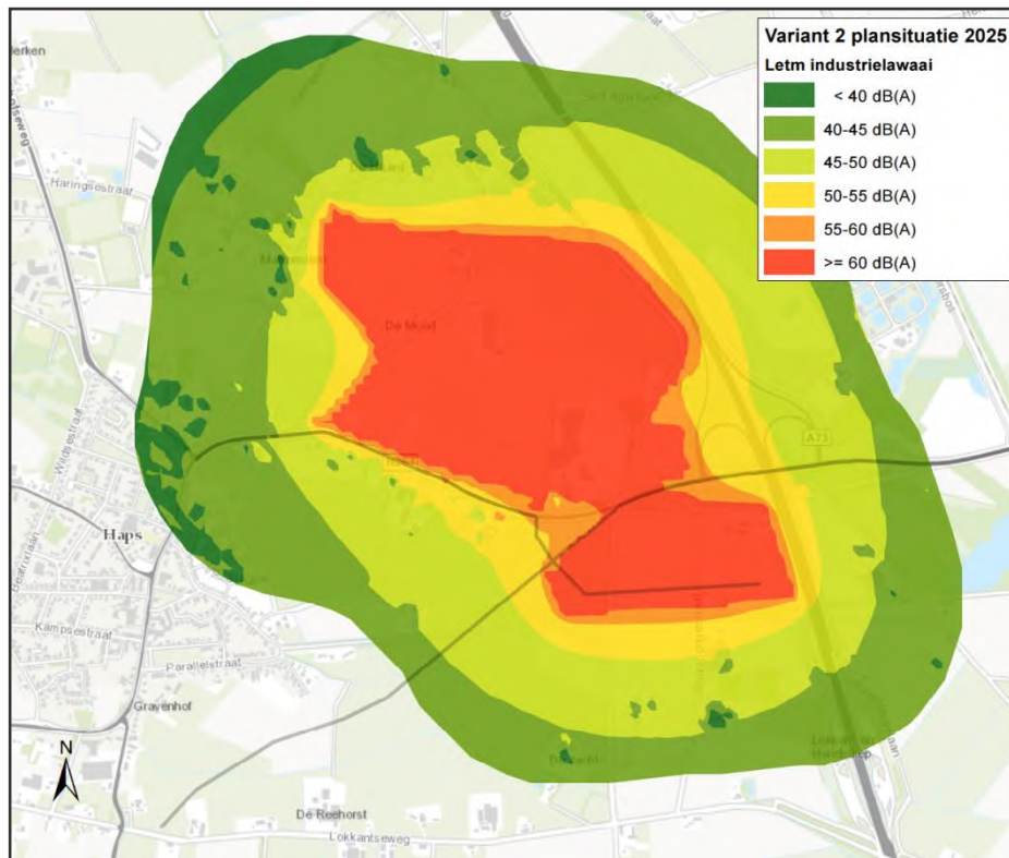
figuur 6.8 Geluidcontouren geluidbelasting L_{etm} industrie plansituatie variant 2 2025
