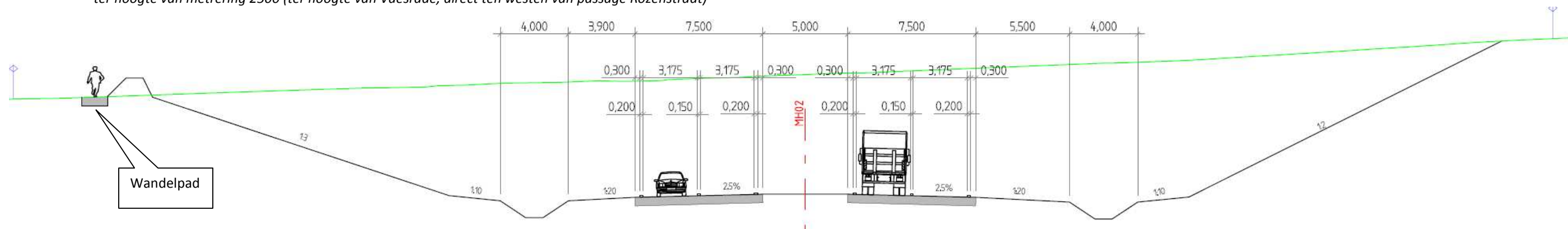
Figuur 3.2 Dwarsprofielen Verdiepte ligging BPL ter hoogte van Vaesrade (MNO Vervat, 2013)
