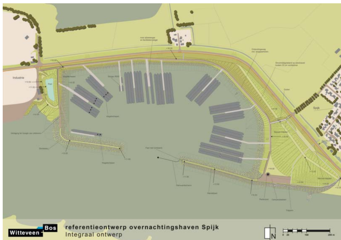
Figuur 2 Schetsontwerp voorkeursvariant Spijk
