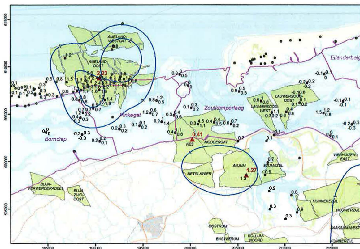
Figuur 3.1: Totale diepe bodemdaling (cm) in Waddenzee en Lauwersmeer door gaswinning in 2009 sinds de nulmetingen in 2006. In blauw de contouren van de gemodelleerde bodemdaling volgens het oude model. De waarden op Ameland betreffen oppervlakte dalingen (zowel diepe als ondiepe dalingen)
