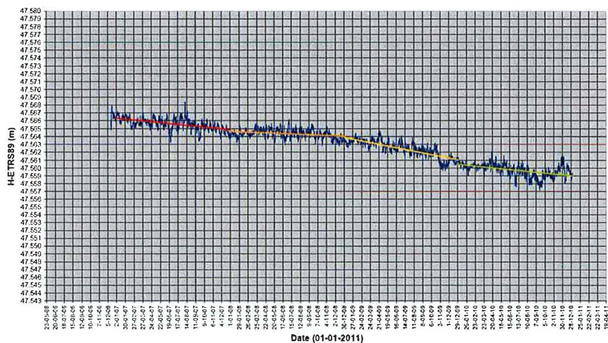
Figuur 3.3: Continue GPS-registraties op de locaties Anjum en Moddergat gestart in 2006 boven het snelst dalende gedeelte van de dalingschotel.
