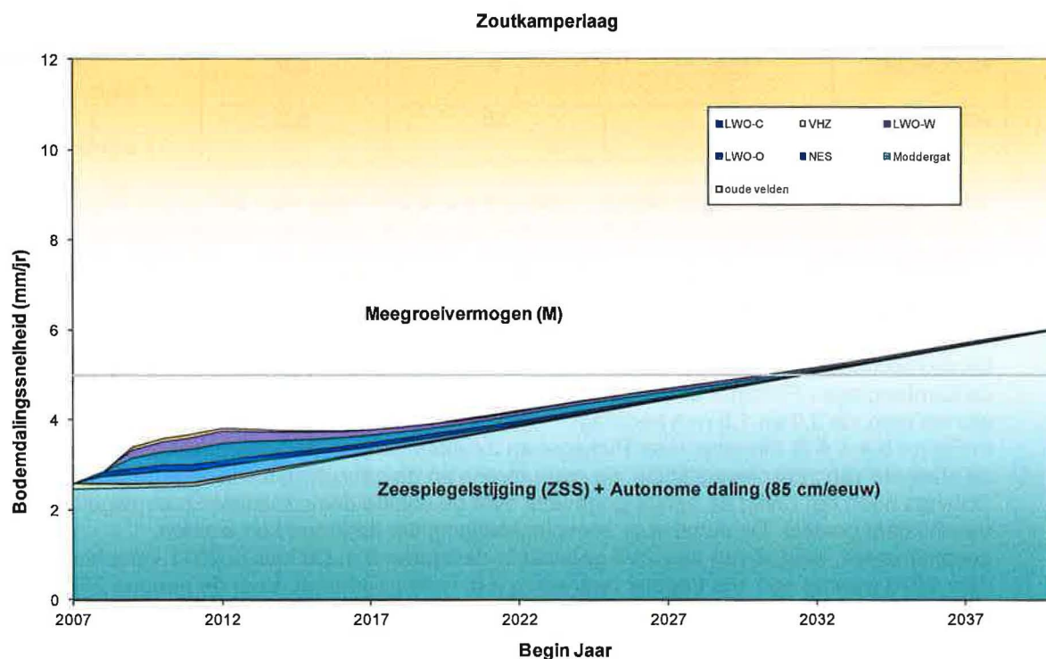
Figuur 3.4B. Bodemdalingsnelheid in de Zoutkamperlaag (6-jaarlijks gemiddelde; "moving average") door gaswinning uit de Ameland- en waddenvelden (MLV) samen met het (in 2006) verwachte zeespiegelstijgingsscenario.
