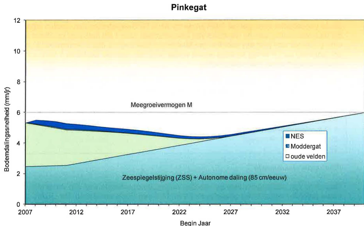
Figuur 3.4A. Bodemdalingssnelheid in het Pinkegat (6-jaarlijks gemiddelde; "moving average") door gaswinning uit de Ameland- en waddenvelden (MLV) samen met het (in 2006) verwachte zeespiegelstijgscenario.
