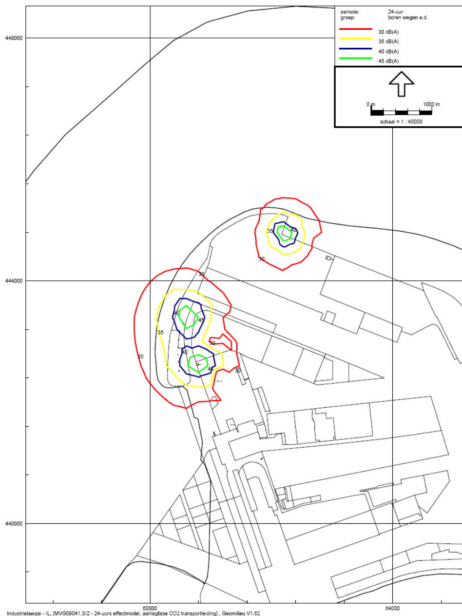
Overzicht van de berekende geluidscontouren vanwege het average boren van kruisingen met wegen e.d.
