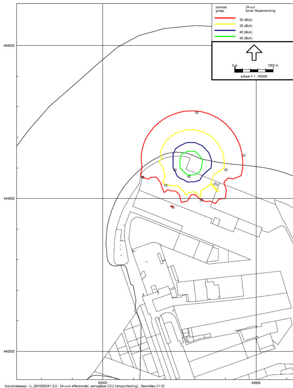
Overzicht van de berekende geluidscontouren vanwege de HDD-boring ten behoeve van de Maasmonding
