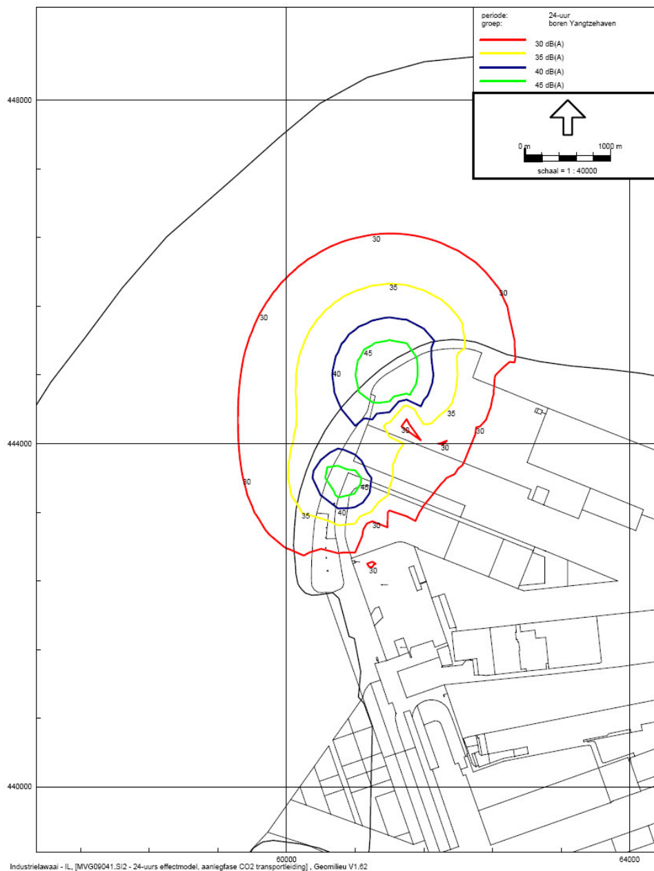
Overzicht van de berekende geluidscontouren vanwege de HDD-boring ten behoeve van de Yangtzehaven
