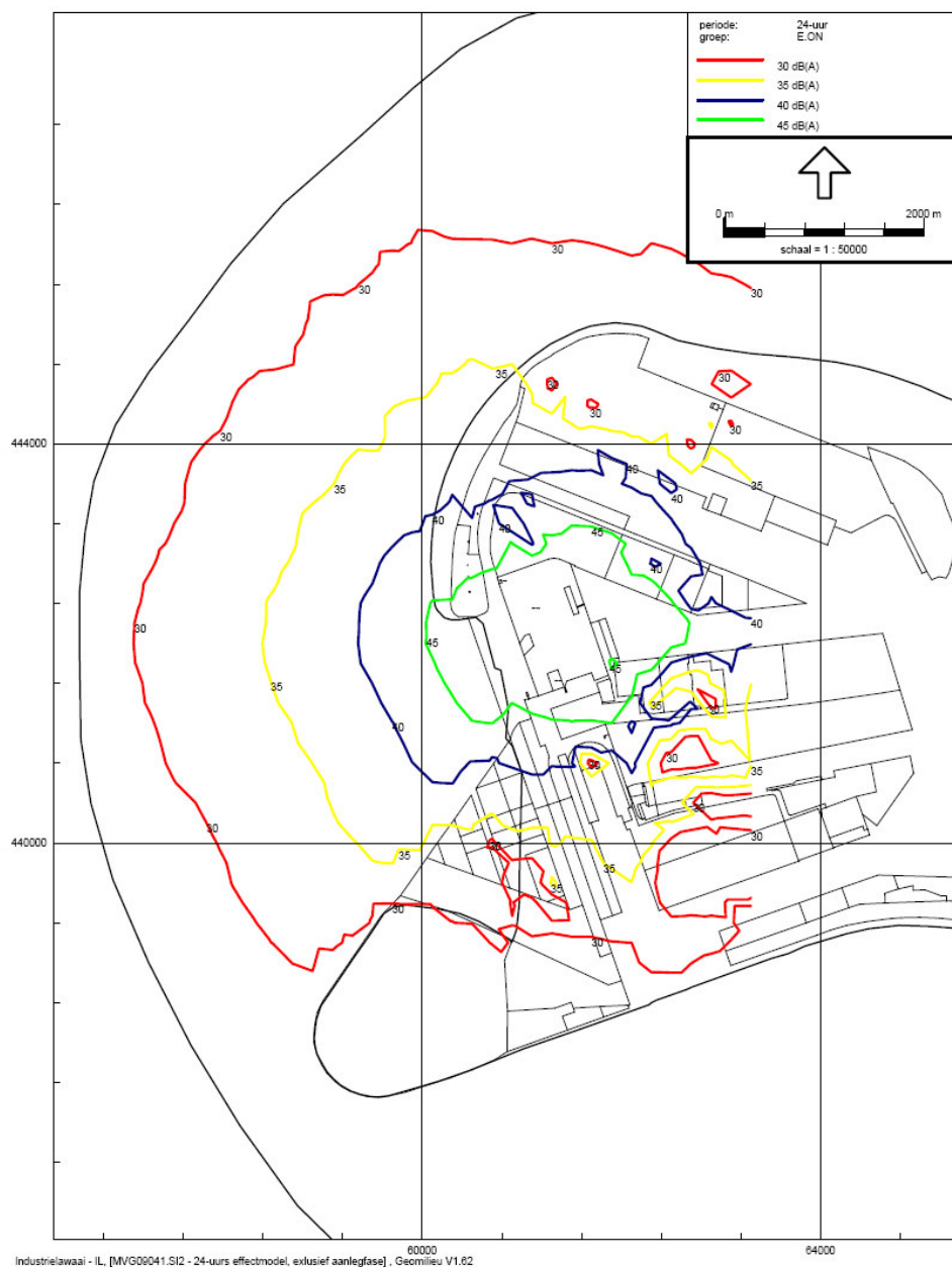
Overzicht van de berekende geluidscontouren vanwege de exploitatie van E.ON, MPP 1 t/m 3, WKC en afvanginstallatie
