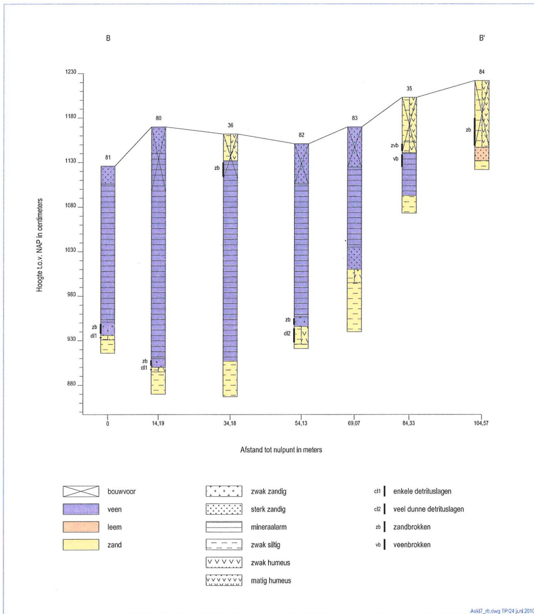
Figuur 3. Dobbe/veentje IV: profiel boorraai B-B'.
