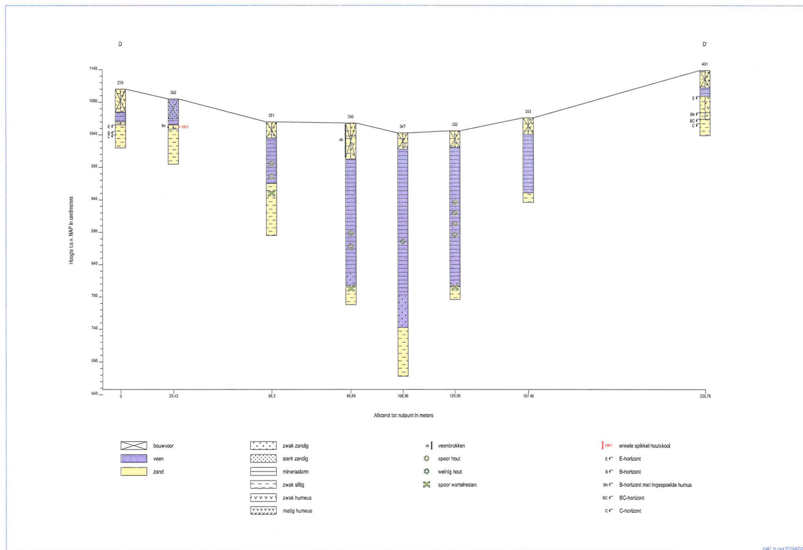
Figuur 5. Dobbe/veentje V: profiel boorrai D-D'.
