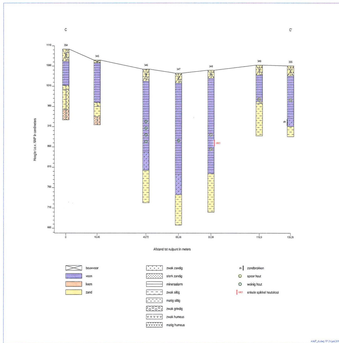
Figuur 4. Dobbe/veentje V: profiel boorraai C-C'.
