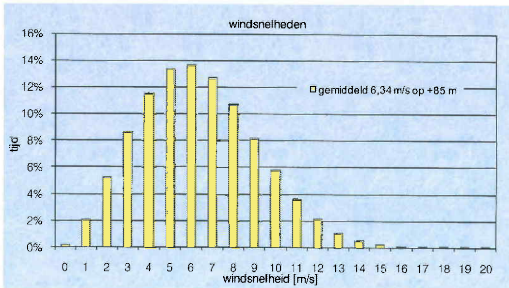
Atbeelding 1-1: windaanbod.
