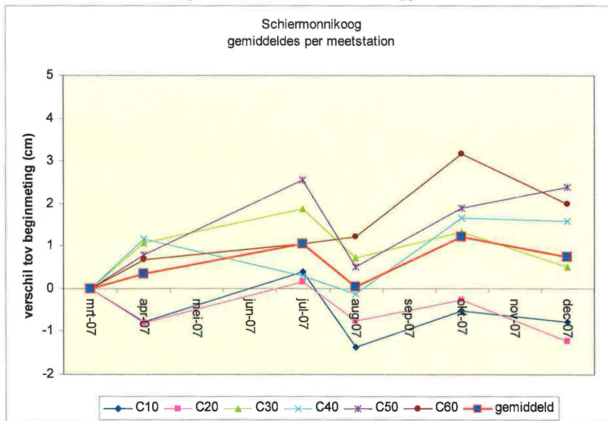
Figuur 14. Gemiddelde meetlijnen van de meetstations C10 tm C60 in het onderzoeksgebied Schiermonnikoog. Tevens is het gemiddelde van deze 6 meetlijnen genomen als weergave van de sedimentatie van het gebied waarin de meetstations liggen.
