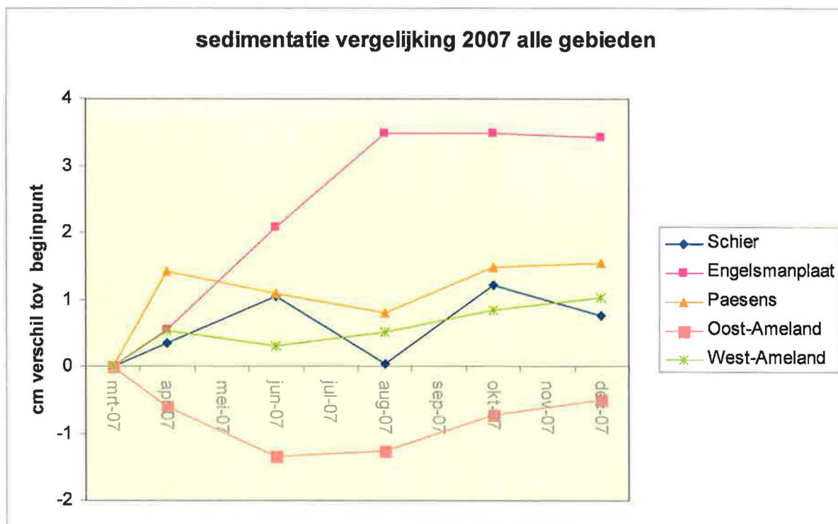
Figuur 20. Onderlinge vergelijking van de sedimentatie in 2007 van de vijf onderzoeksgebieden.
