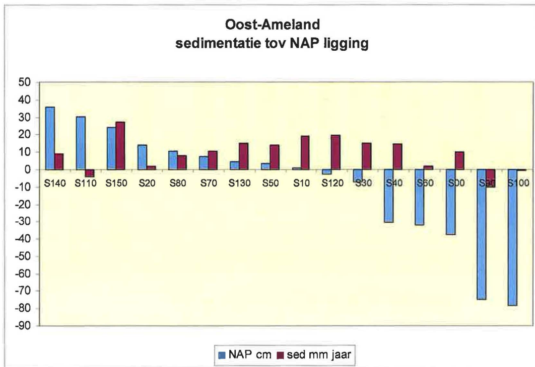
Figuur 21. Wadsedimentatie ten opzichte van hoogte ligging van de meetstations bij Oost-Ameland. Sedimentatiesnelheid in mm per jaar over de totale meetperiode. Meetperiode varieert van 3 tot 7 jaar tussen 2000 en 2007 (zie tabel 1). Meetdatum december 2007.
