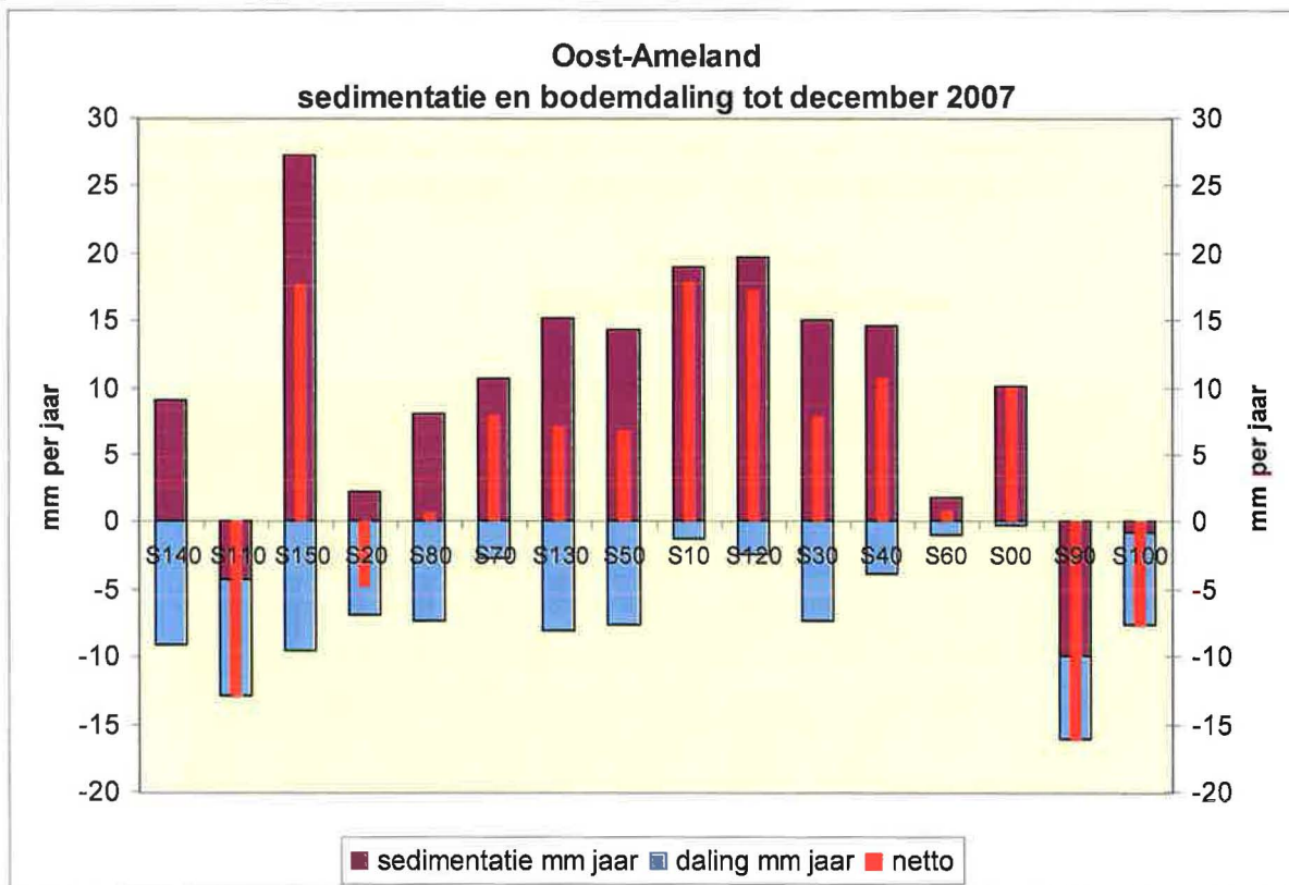
Figuur 22. Netto gemiddelde sedimentatie/erosie per jaar gedurende de gehele meetperiode per meetstation. Bijgewerkt tm december 2007.
