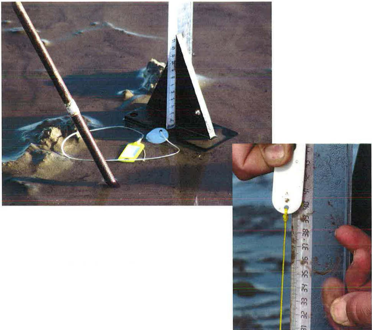
Foto 4. Meetlineaal met meetvoet. Deze wordt steeds op dezelfde wijze op de bodem gezet waarna de lengte van het meettouw langs de schaal wordt afgelezen.
