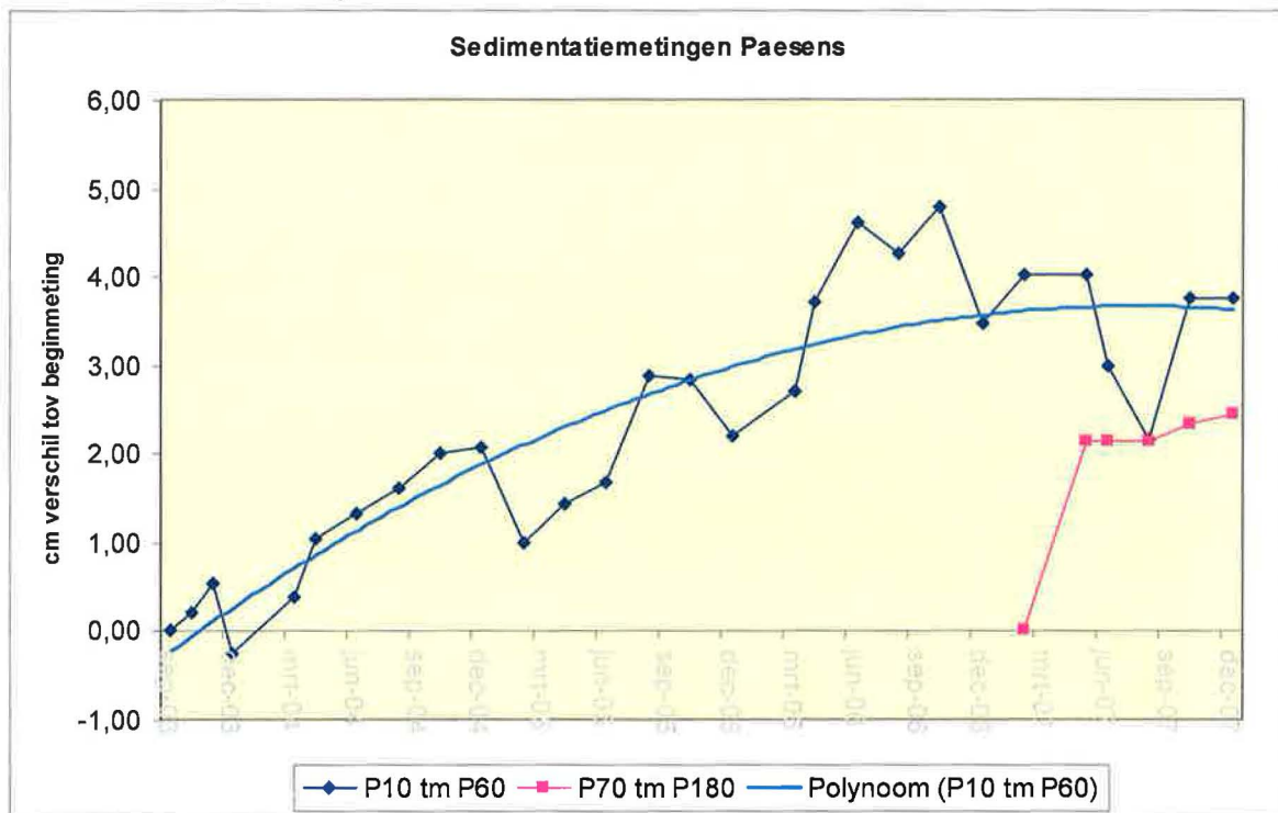
Figuur 11. Gemiddelde van de gemiddeldes van meetstations P10 tm P60 en P70 tm P180 in het onderzoeksgebied bij Paesens.
