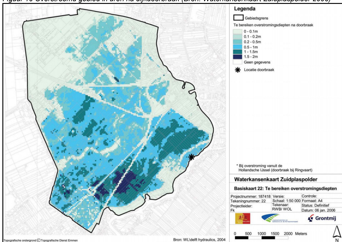
Figuur 11 Overstromingsdiepten na 120 uur (Bron: Waterkansenkaart Zuidplaspolder 2006)
