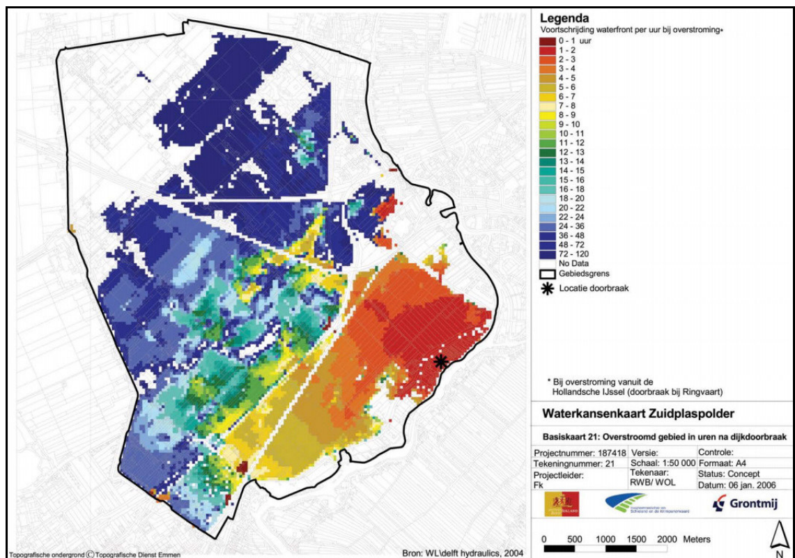
Figuur 10 Overstroomd gebied in uren na dijkdoorbraak (Bron: Waterkansenkaart Zuidplaspolder 2006)
