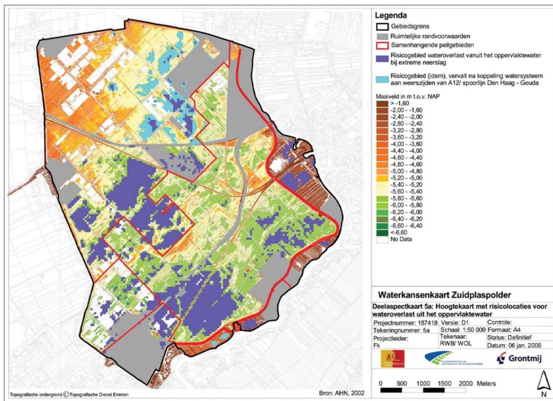
Figuur 15 risicolocaties wateroverlast (Bron: Waterkansenkaart Zuidplaspolder 2006)
