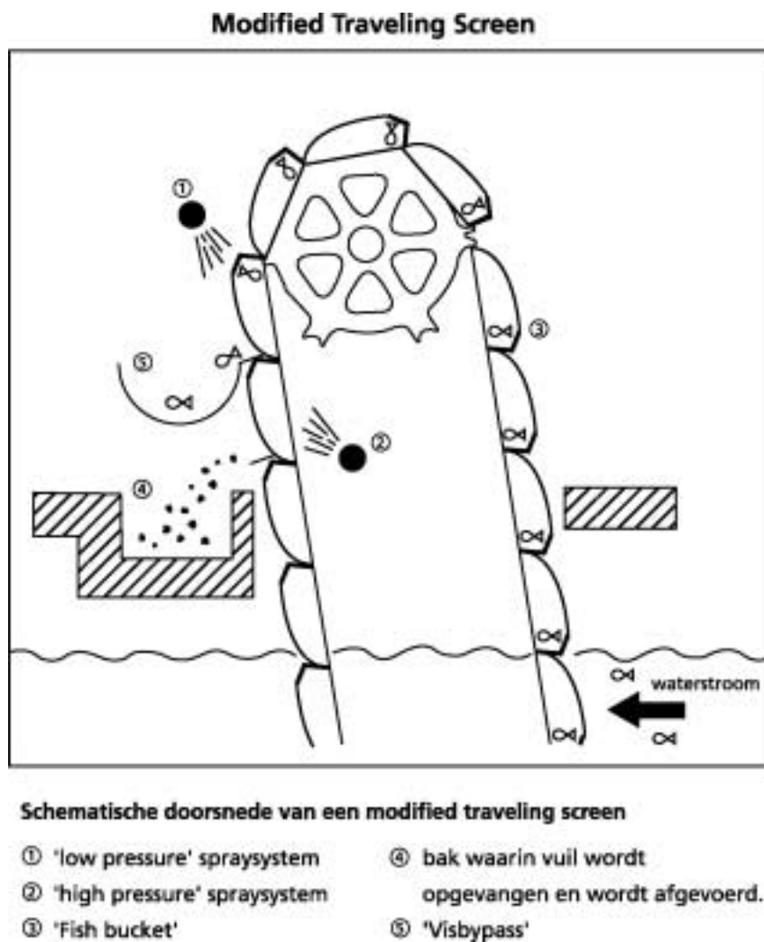
Figuur 3.3 Schematisch zijaanzicht van een 'flow-through' modified traveling screen
