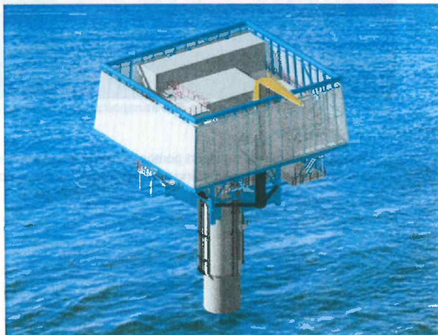
Transformatorstation (voorbeeld)
