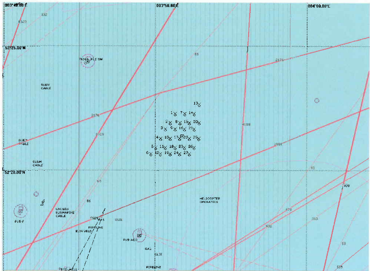
Figuur A1-1 Windpark Rijnvel Noord, basis variant met 27 windturbines van 3 MW
