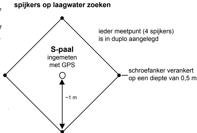
Figuur 1 Bovenaanzicht van een meetpunt. Ieder meetpunt bestaat uit 4 schroefankers en wordt gemarkeerd door een S-paal. Om de kans op verlies van gegevens ten gevolge van het verdwijnen van schroefankers te minimaliseren, is op iedere meetlocatie een alternatief meetpunt ingericht (A-paal) 10 meter ten noorden van de S-paal.
