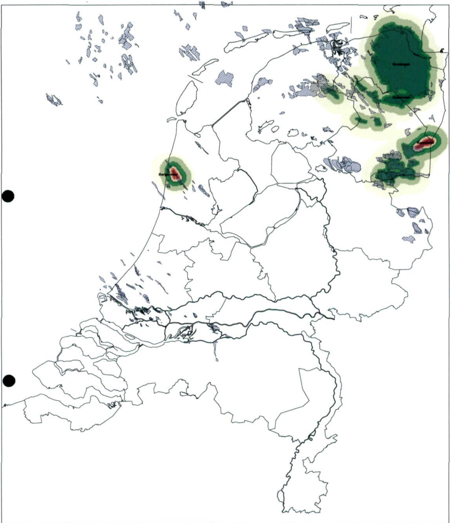
Pieksnelheid op de fundering (T = 100)
