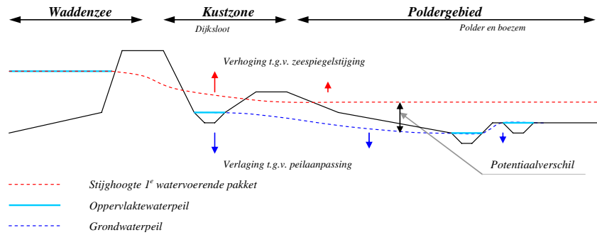
Figuur 5-1 Dwarsprofiel noord-zuid ten westen van het Lauwersmeer.
