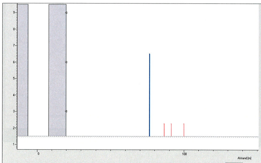
Schermdoelgebied 3, ten behoeve van cluster 1-4 maaiveld (worst-case)
