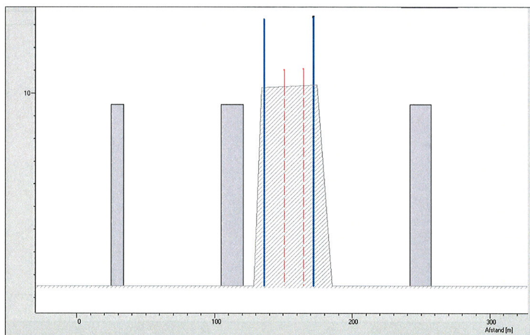
Schermdoelgebied 2, ten behoeve van cluster 7 en 14
