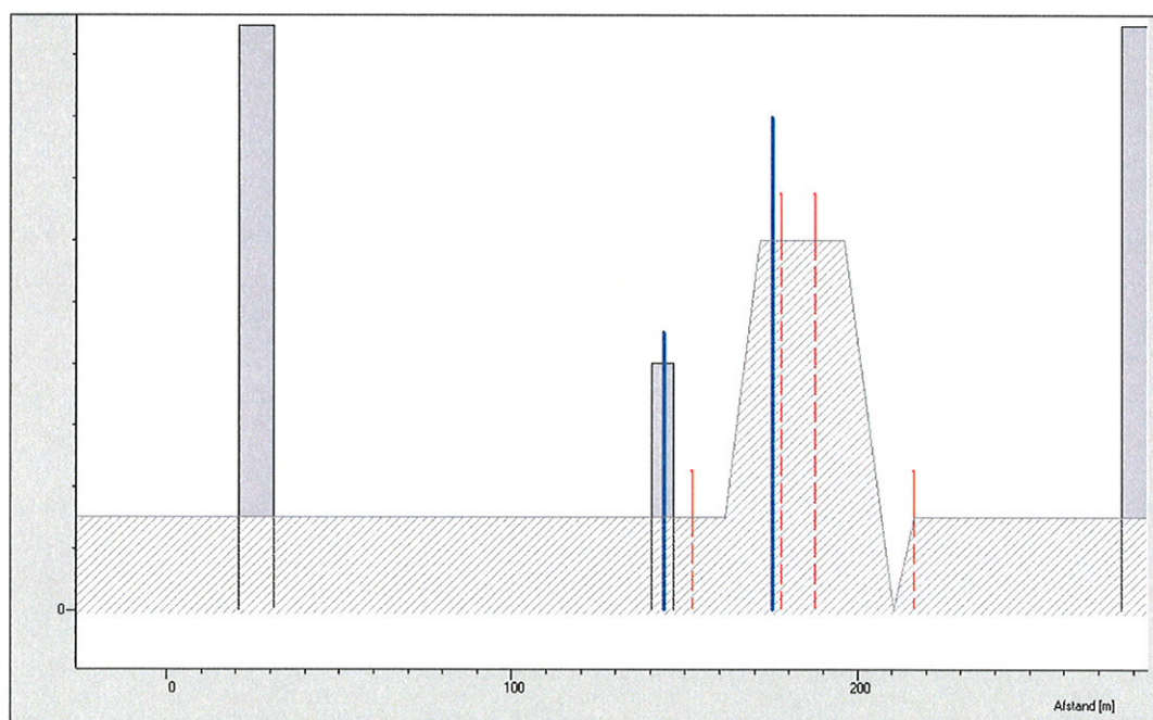
Schermdoelgebied 3, ten behoeve van cluster 2-3 verhoogd (worst-case)
