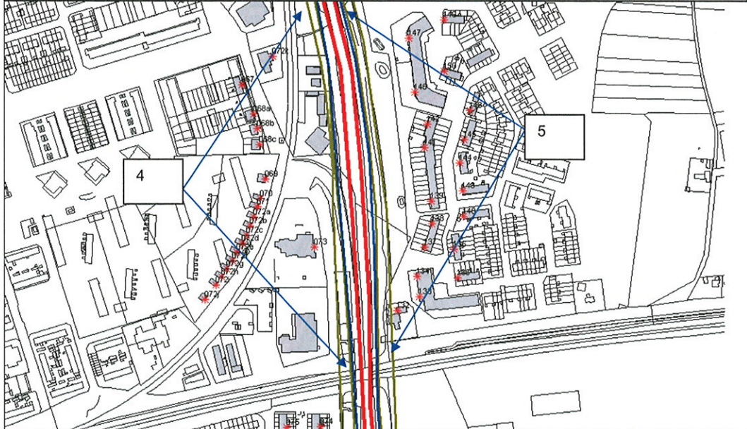
Schermdoelgebied 2, ten behoeve van cluster 8-9 en 12
