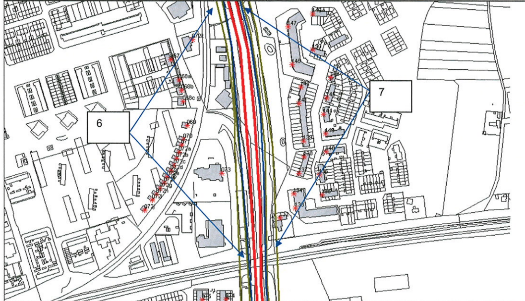
Schermdoelgebied 2, ten behoeve van cluster 8-9 en 13
