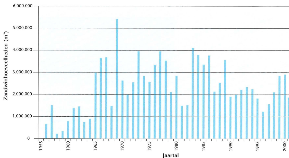
Figuur 15 Zandwinhoeveelheden in de Westerschelde.
