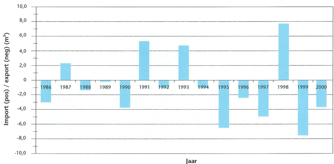
Figuur 18 Zandimport/export vanuit de Westerschelde.
