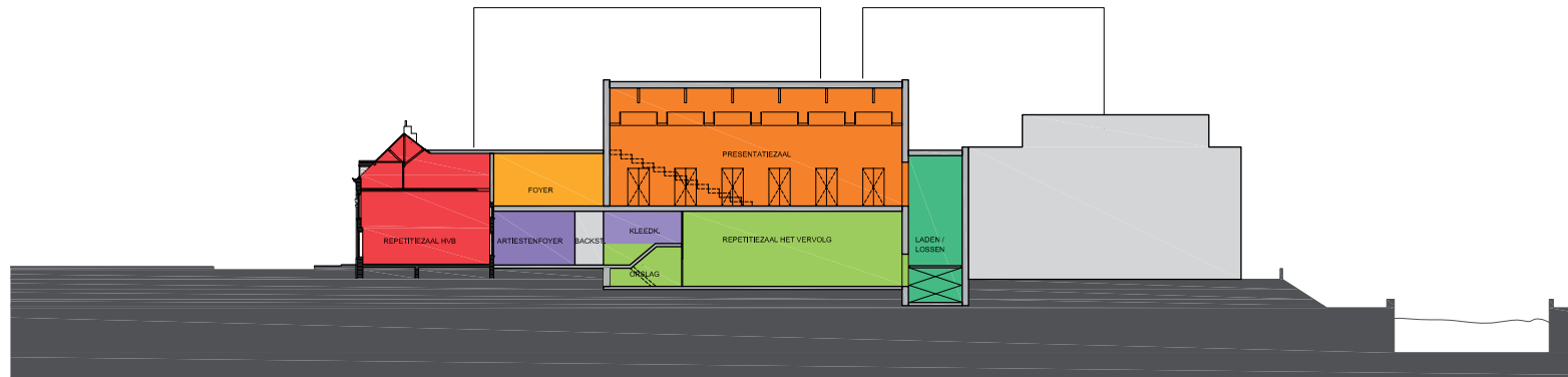
DOORSNEDE E-E
