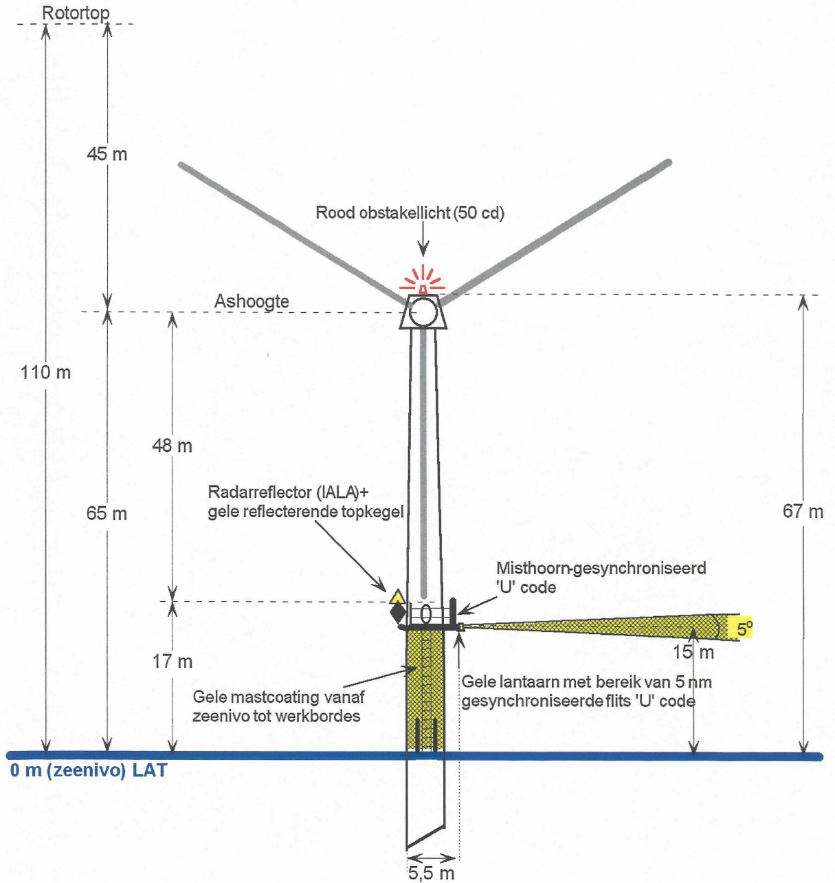
FIGUUR 1 VERLICHTINGSPLAN SCHEEP- EN LUCHTVAART WINDTURBINES OFFSHORE WINDPARK (according IALA Recommendation)
