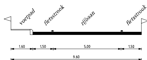
Principeprofiel zijweg met fietsstroken
