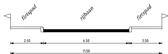
Principeprofiel zijweg met aanliggende fietspaden
